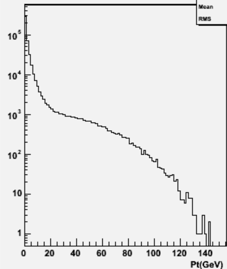
Start point Z : w101578 n3n3cse1n1_o
