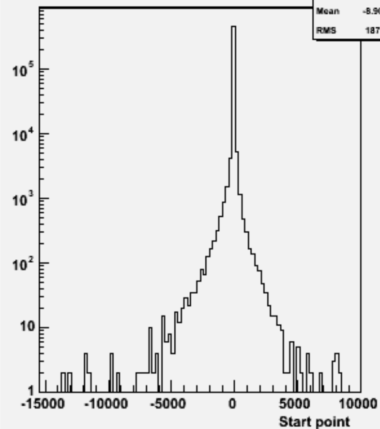
Start point Z : w101578 n3n3cse1n1_o
