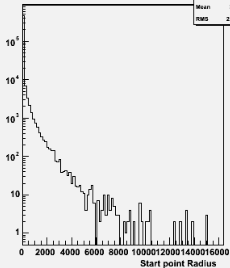
Start point R : w101578 n3n3cse1n1_o
