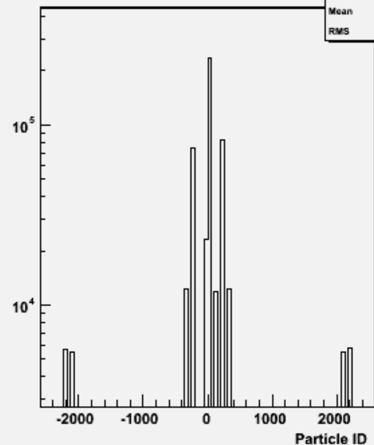
Particle ID : w101576 n3n3cse1n1_o
