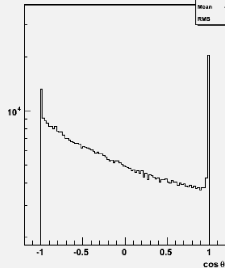
Particle \cos\theta : w101576 n3n3cse1n1_o
