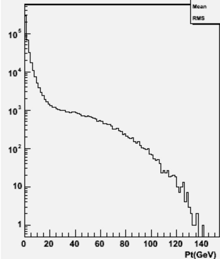
Particle Pt : w101576 n3n3cse1n1_o
