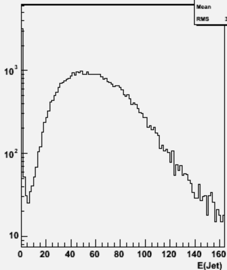
Jet energies(All jets)w101573 n3n3udsc_o
