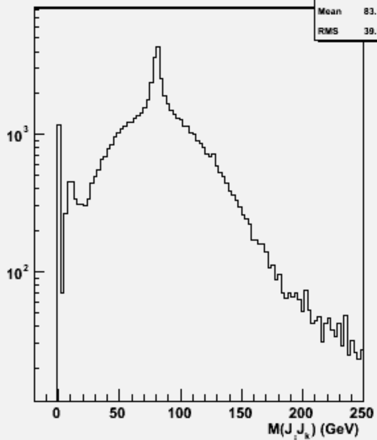
2jets mass(All comb)w101573 n3n3udsc_o
