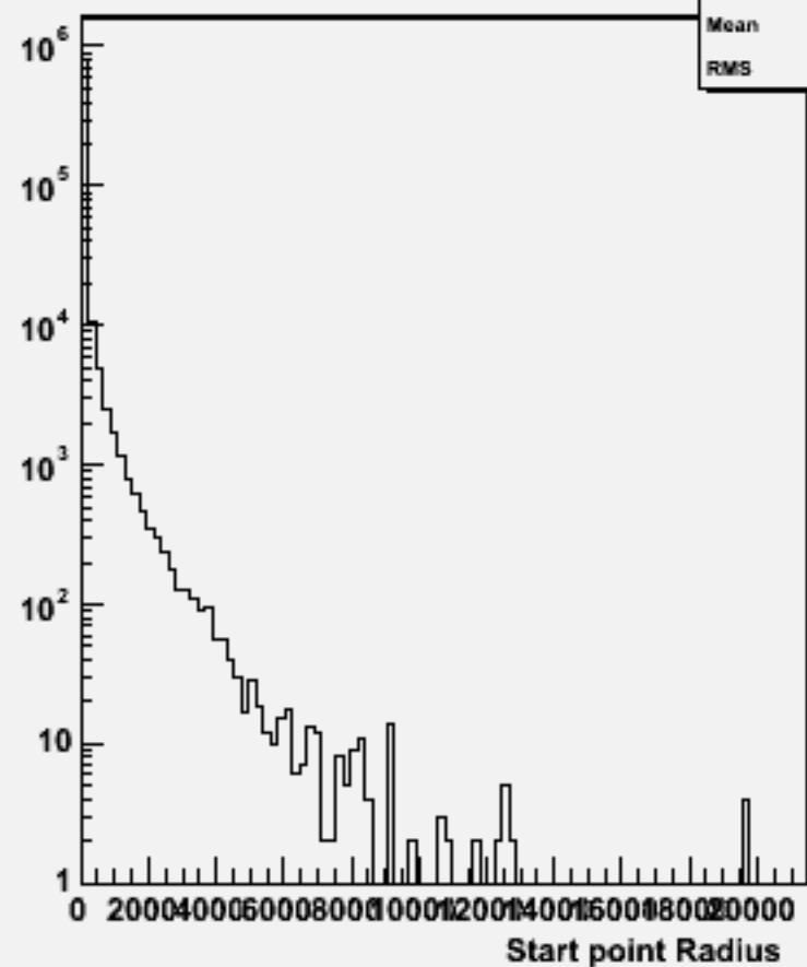
Start point R : w101573 n3n3udsc_o
