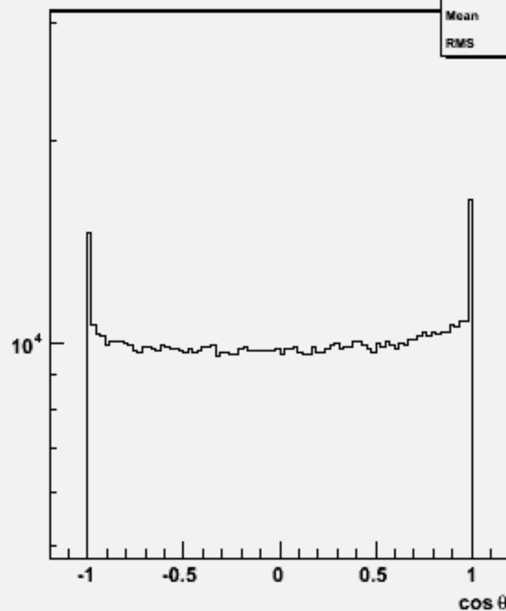
Particle cos \theta : w101573 n3n3udsc_o
