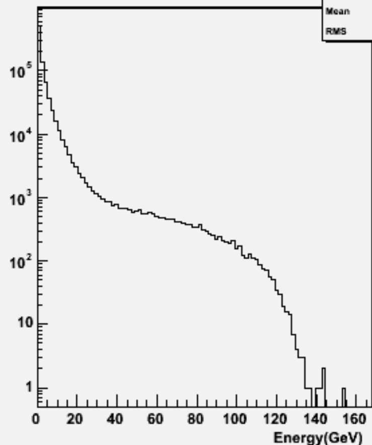
Particle Energy : w101573 n3n3udsc_o
