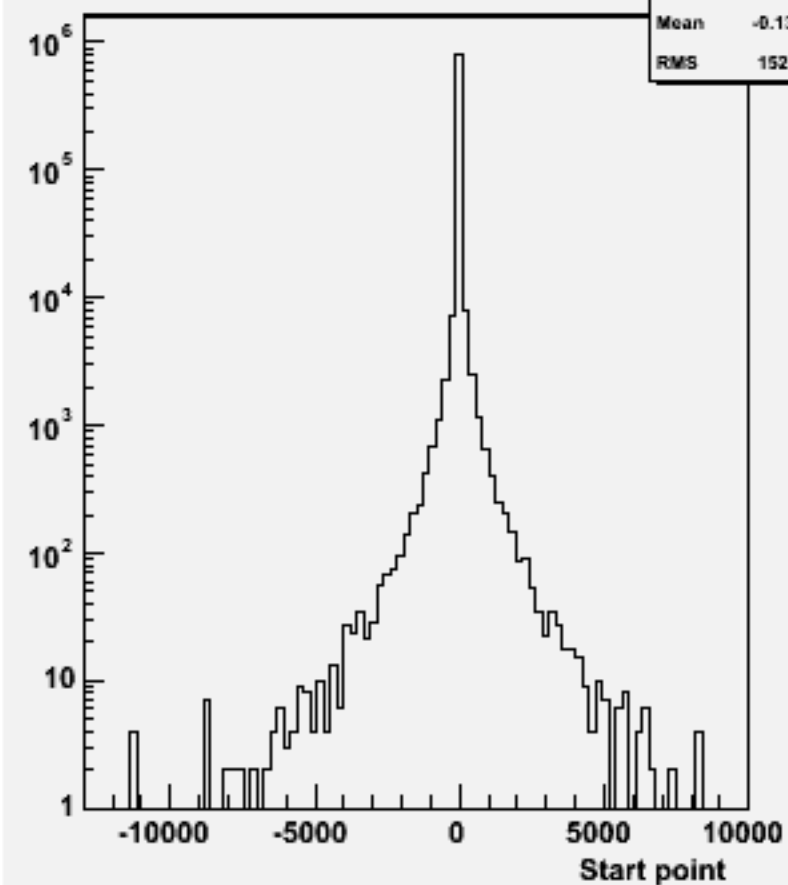
Start point Z : w101573 n3n3udsc_o
