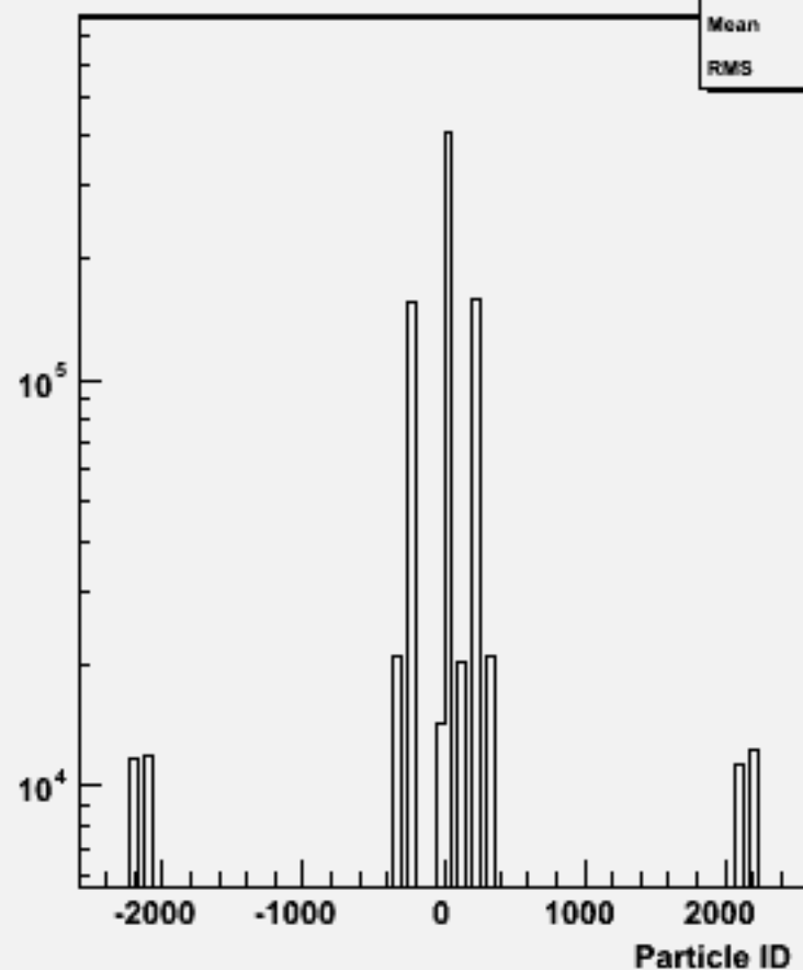
Particle ID : w101573 n3n3udsc_o
