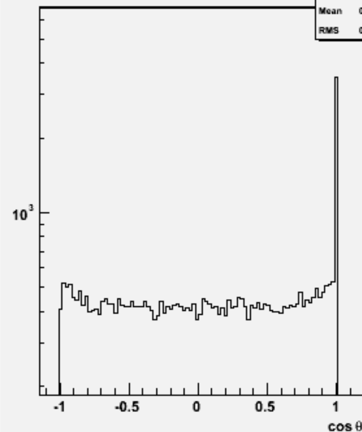
Jet cos \theta (All jets)w101573 n3n3udsc_o
