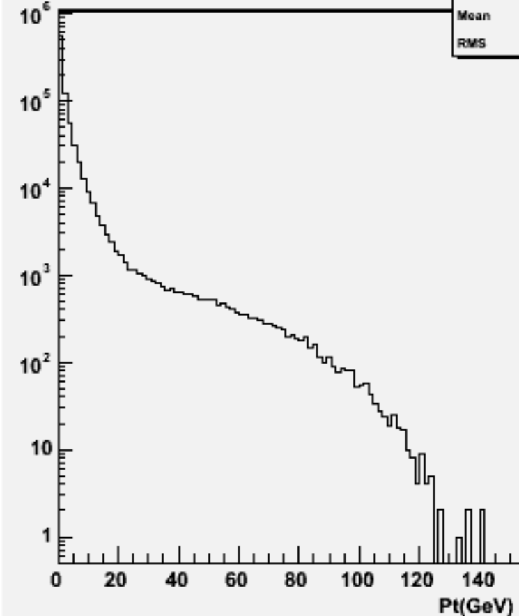
Particle Pt : w101573 n3n3udsc_o
