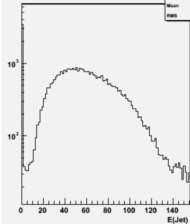
Jet energies(All jets)w101572 n3n3udsc_o
