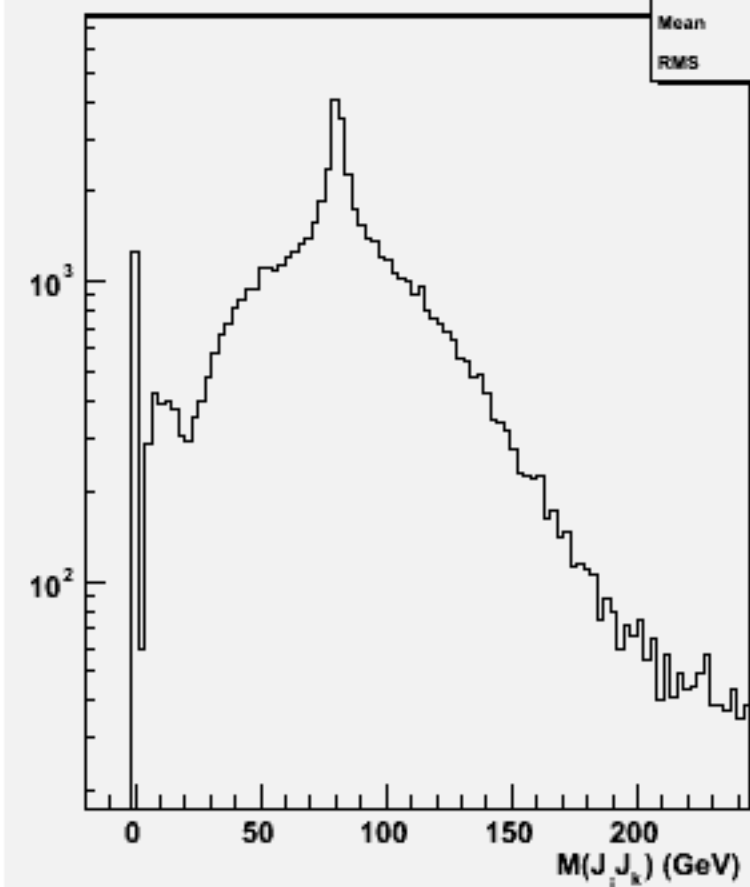
2jets mass(All comb)w101572 n3n3udsc_o
