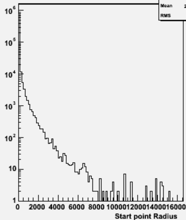
Start point R : w101572 n3n3udsc_o
