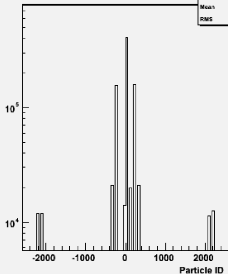
Particle ID : w101572 n3n3udsc_o
