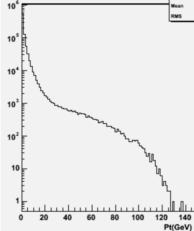
Particle Pt : w101572 n3n3udsc_o
