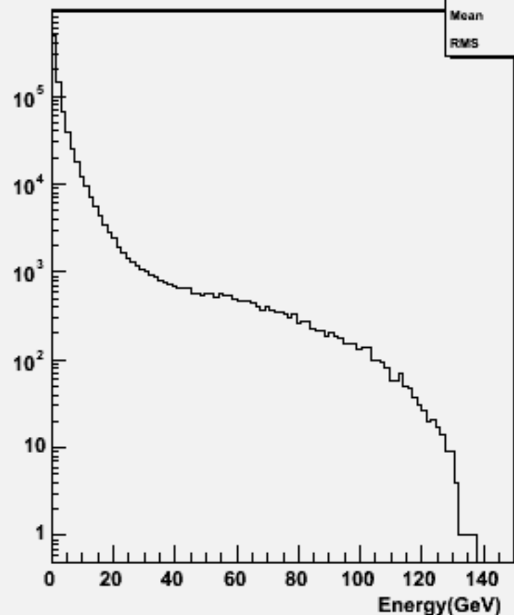
Particle Energy : w101572 n3n3udsc_o
