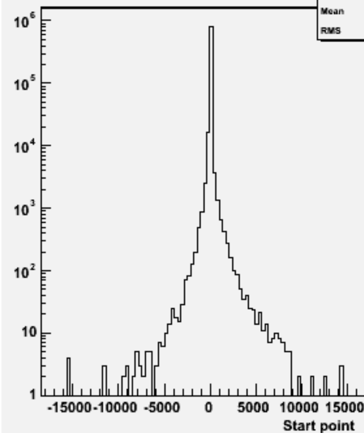
Start point Z : w101572 n3n3udsc_o
