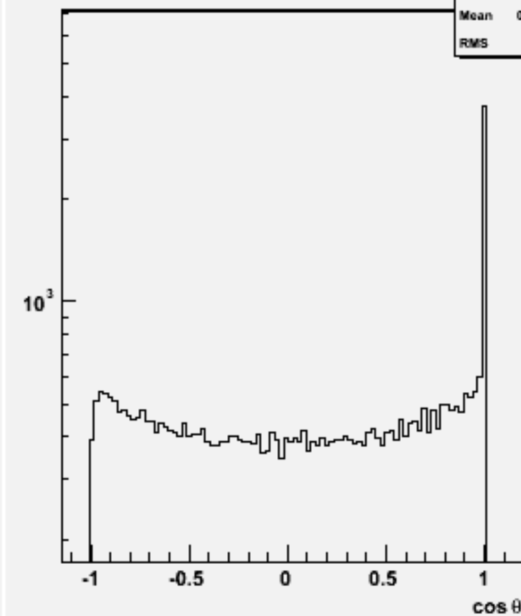
Jet cosθ (All jets)w101572 n3n3udsc_o
