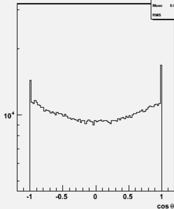
Particle cos \theta : w101572 n3n3udsc_o
