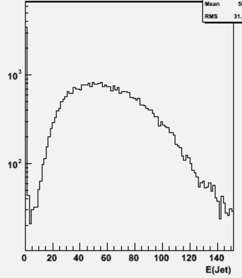
Jet energies(All jets)w101568 n3n3uddu_o
