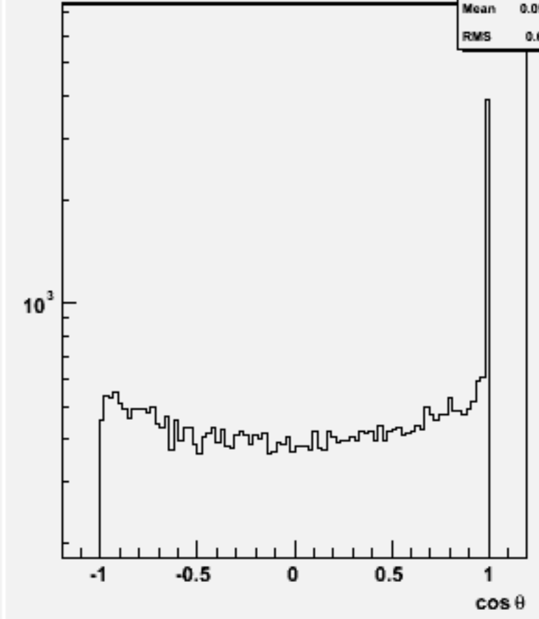
Jet cosθ (All jets)w101568 n3n3uddu_o
