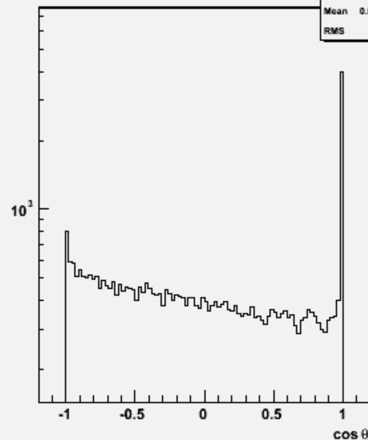
Jet cos \theta (All jets)w101561 n3n3ude2n2_o
