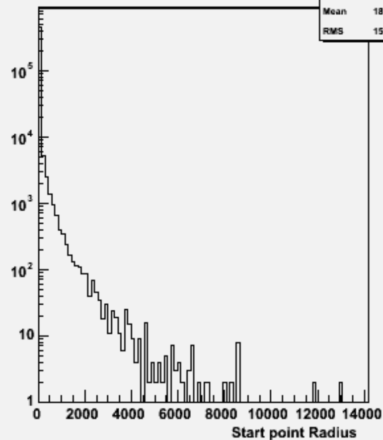
Start point R : w101561 n3n3ude2n2_o
