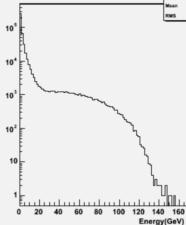
Start point R : w101561 n3n3ude2n2_o
