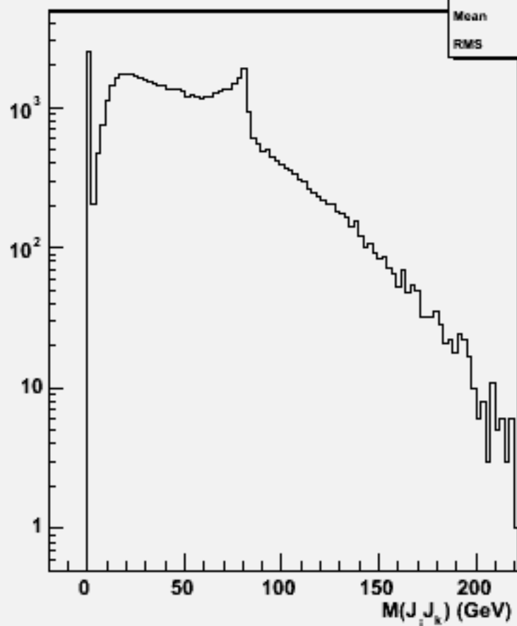
2jets mass(All comb)w101561 n3n3ude2n2_o
