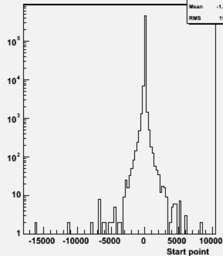
Start point Z : w101561 n3n3ude2n2_o
