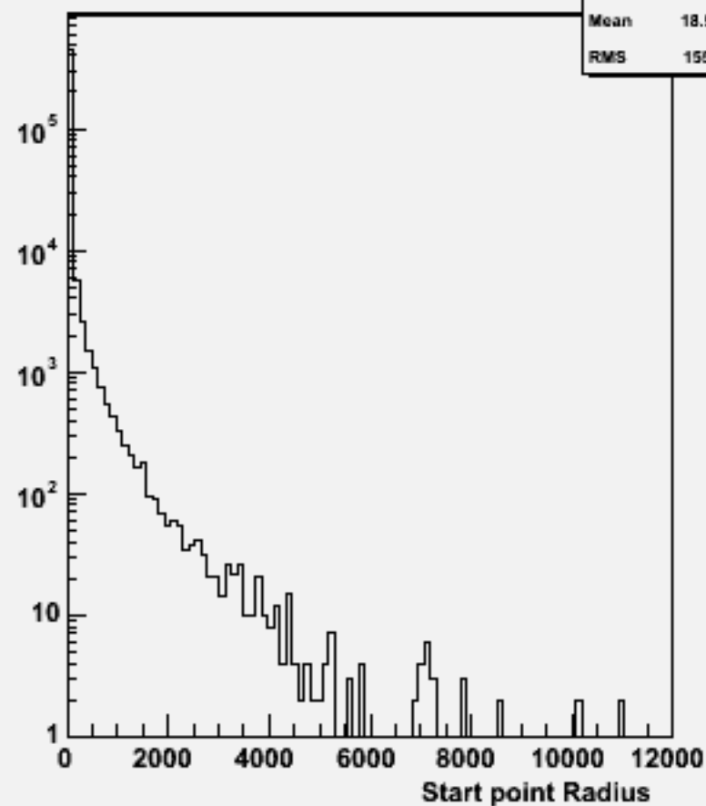
Start point R : w101558 n3n3ude1n1_o
