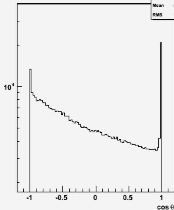
Particle cosθ : w101558 n3n3ude1n1_o
