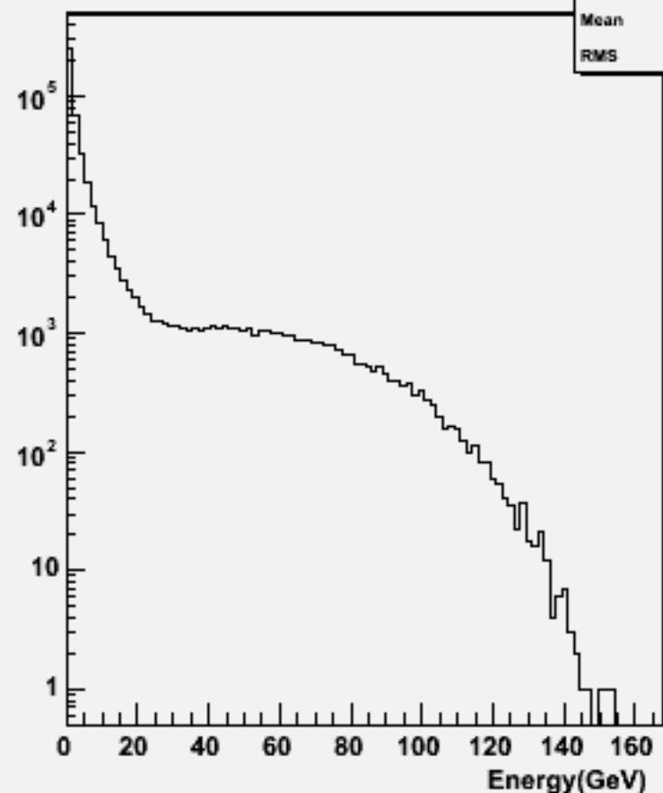
Start point R : w101558 n3n3ude1n1_o
