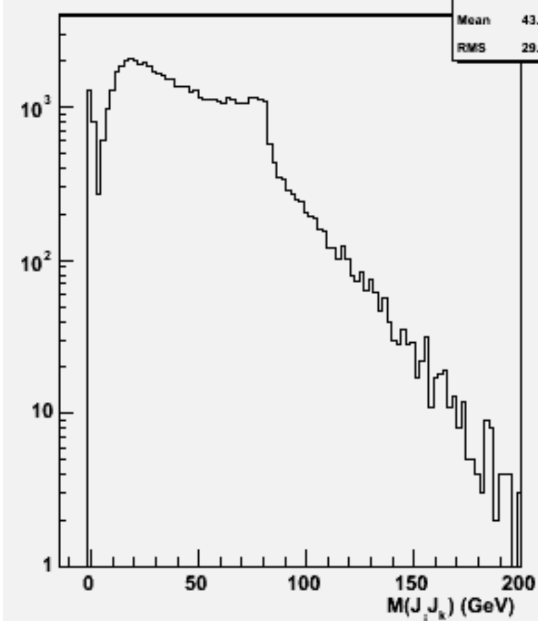
2jets mass(All comb)w101553 n3n3n3e3sc_o
