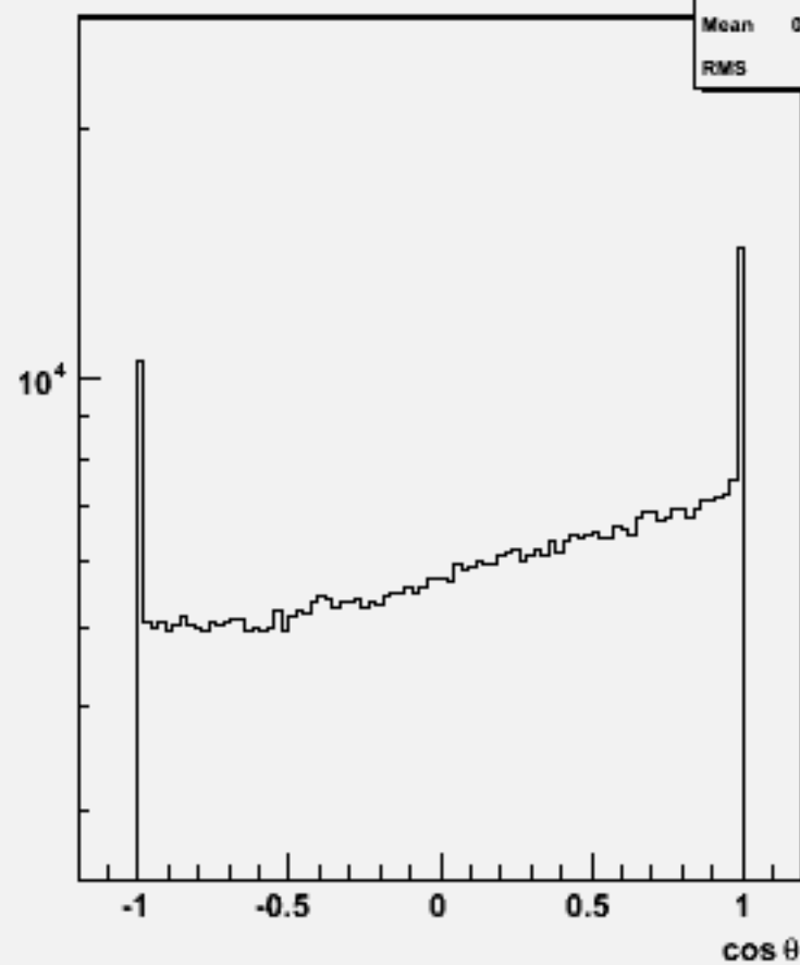
Particle cosθ : w101553 n3n3n3e3sc_o
