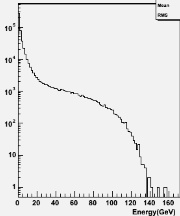
Start point R : w101553 n3n3n3e3sc_o
