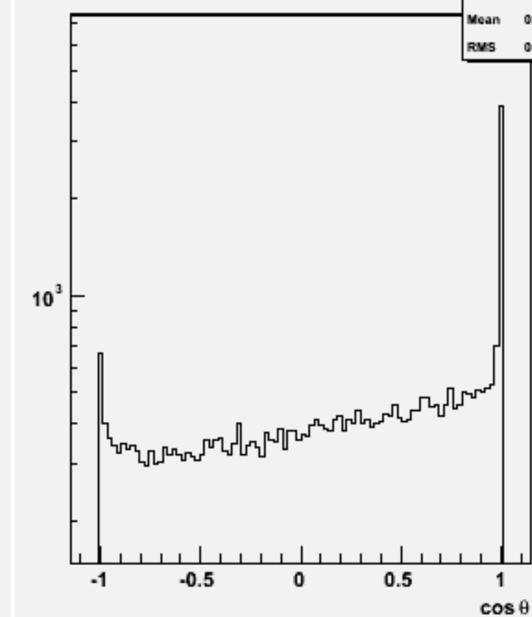
Jet cos \theta (All jets)w101553 n3n3n3e3sc_o
