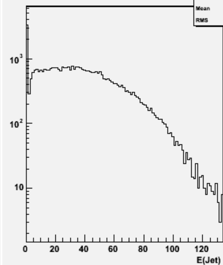
Jet energies(All jets)w101553 n3n3n3e3sc_o
