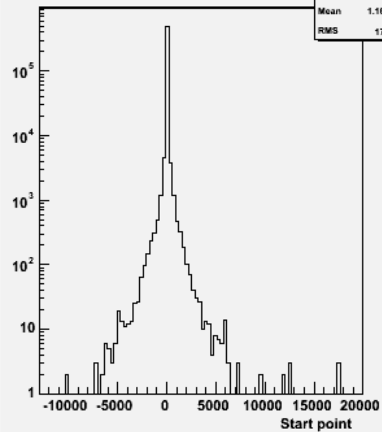
Start point Z : w101553 n3n3n3e3sc_o
