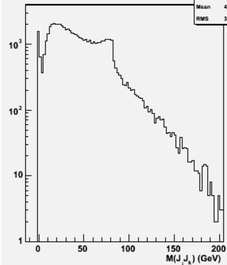
2jets mass(All comb)w101552 n3n3n3e3sc_o
