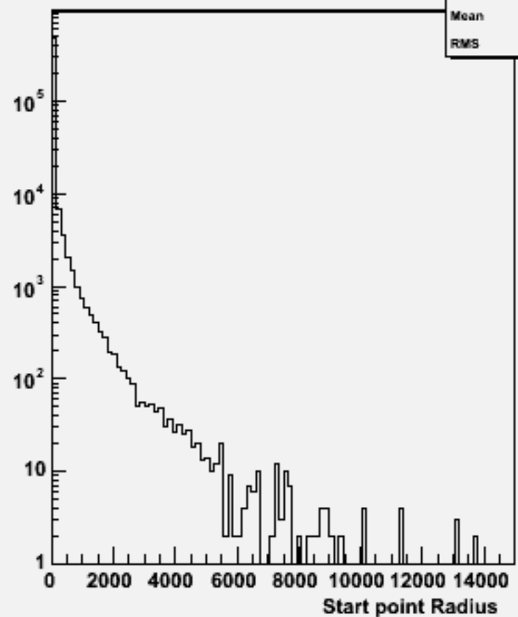
Start point R : w101552 n3n3n3e3sc_o
