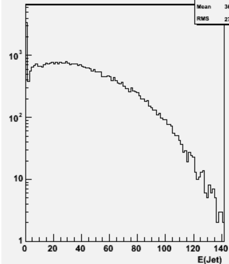
Jet energies(All jets)w101552 n3n3n3e3sc_o
