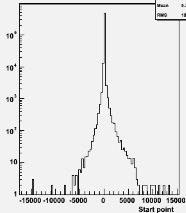
Start point Z : w101552 n3n3n3e3sc_o
