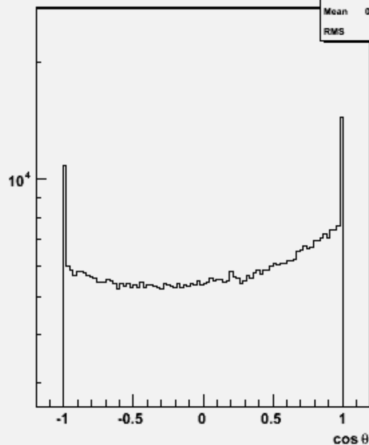
Particle \cos\theta : w101552 n3n3n3e3sc_o
