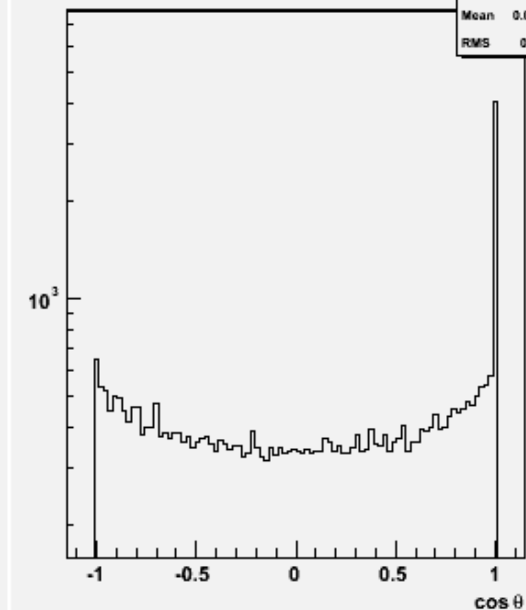
Jet cos \theta (All jets)w101552 n3n3n3e3sc_o
