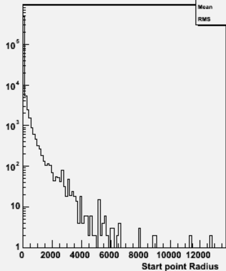
Start point R : w101549 n3n3n3e3du_o
