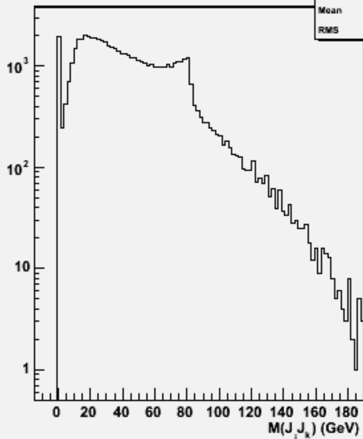
2jets mass(All comb)w101549 n3n3n3e3du_o
