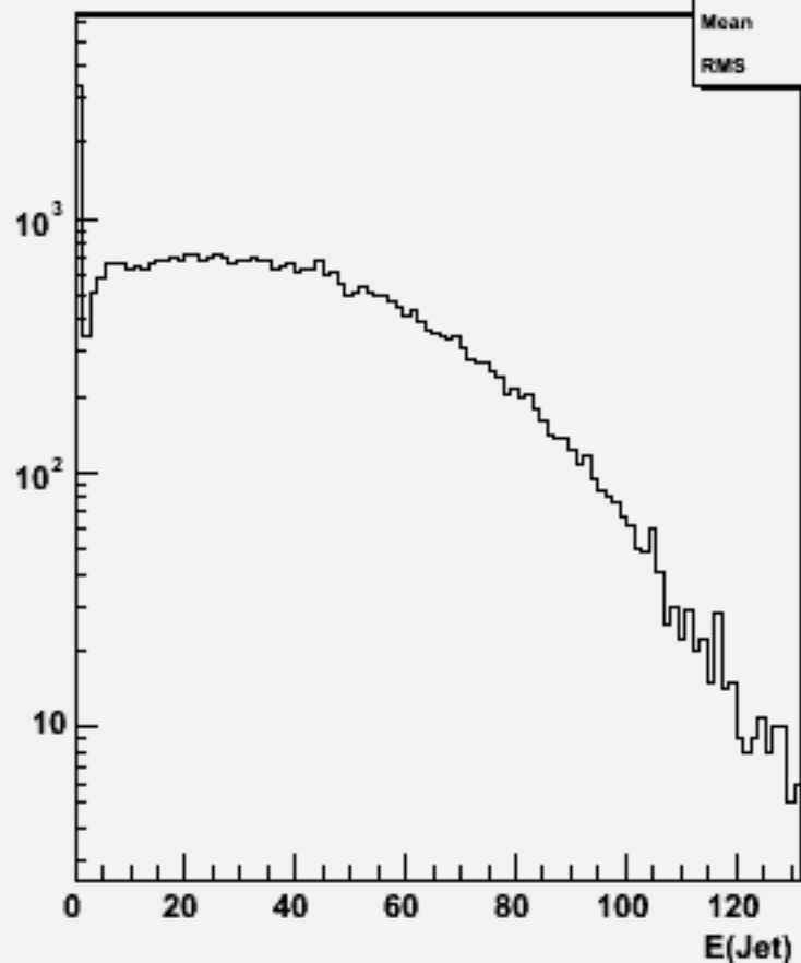
Jet energies(All jets)w101549 n3n3n3e3du_o
