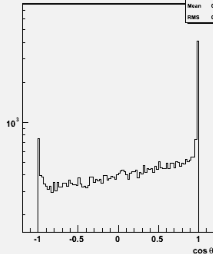
Jet cos \theta (All jets)w101549 n3n3n3e3du_o
