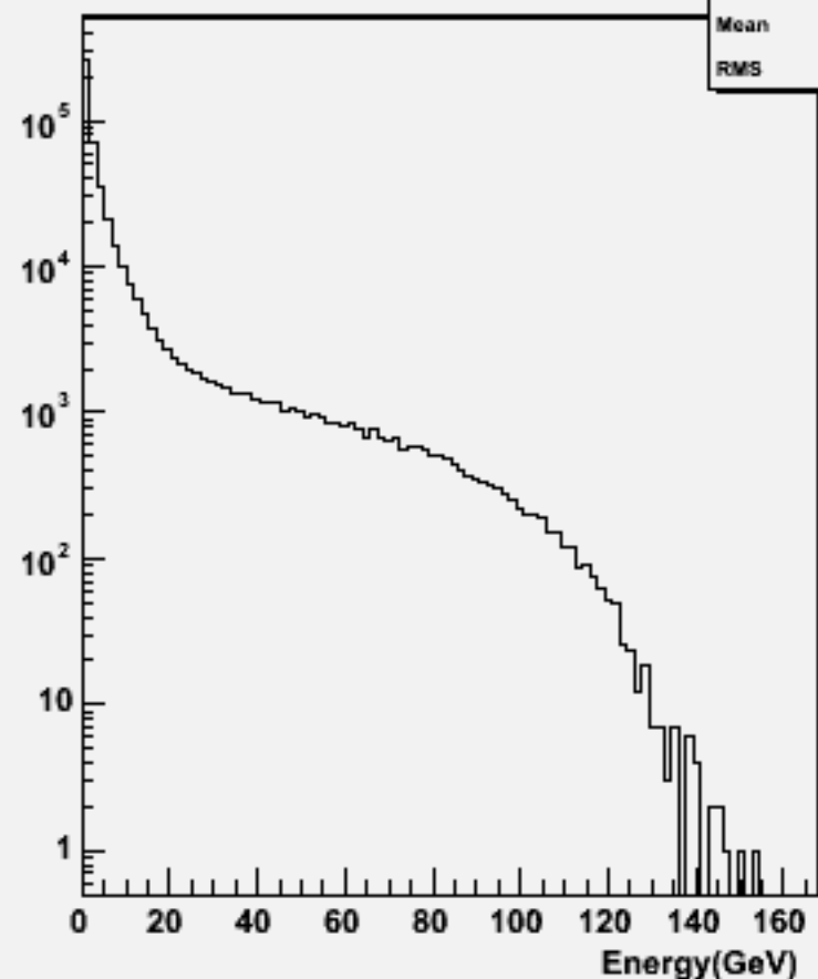
Start point R : w101549 n3n3n3e3du_o
