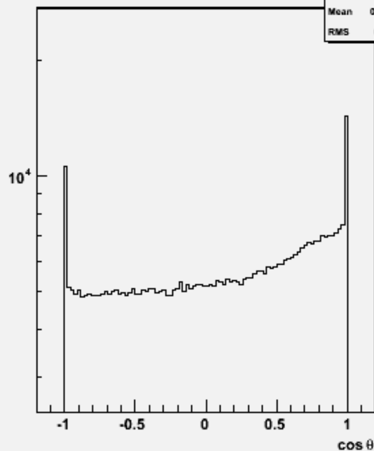
Particle cos \theta : w101532 n3n3n2e2sc_o
