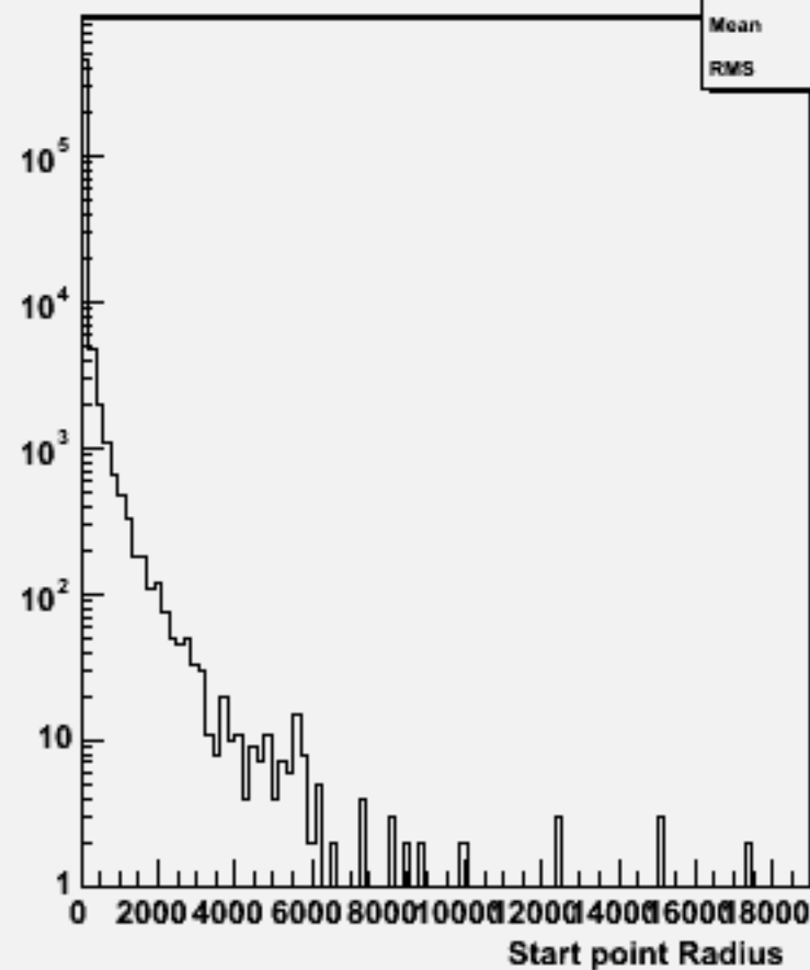
Start point R : w101529 n3n3n2e2du_o
