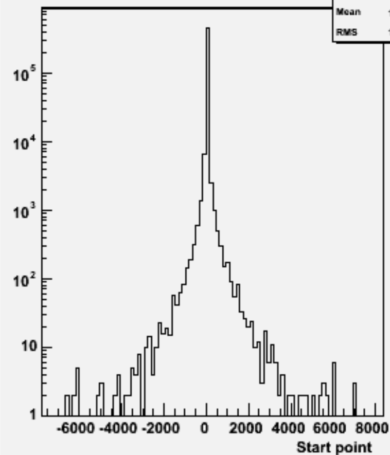
Start point Z : w101529 n3n3n2e2du_o
