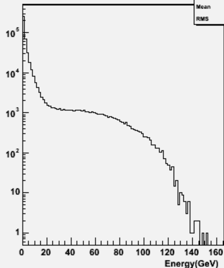
Start point R : w101529 n3n3n2e2du_o
