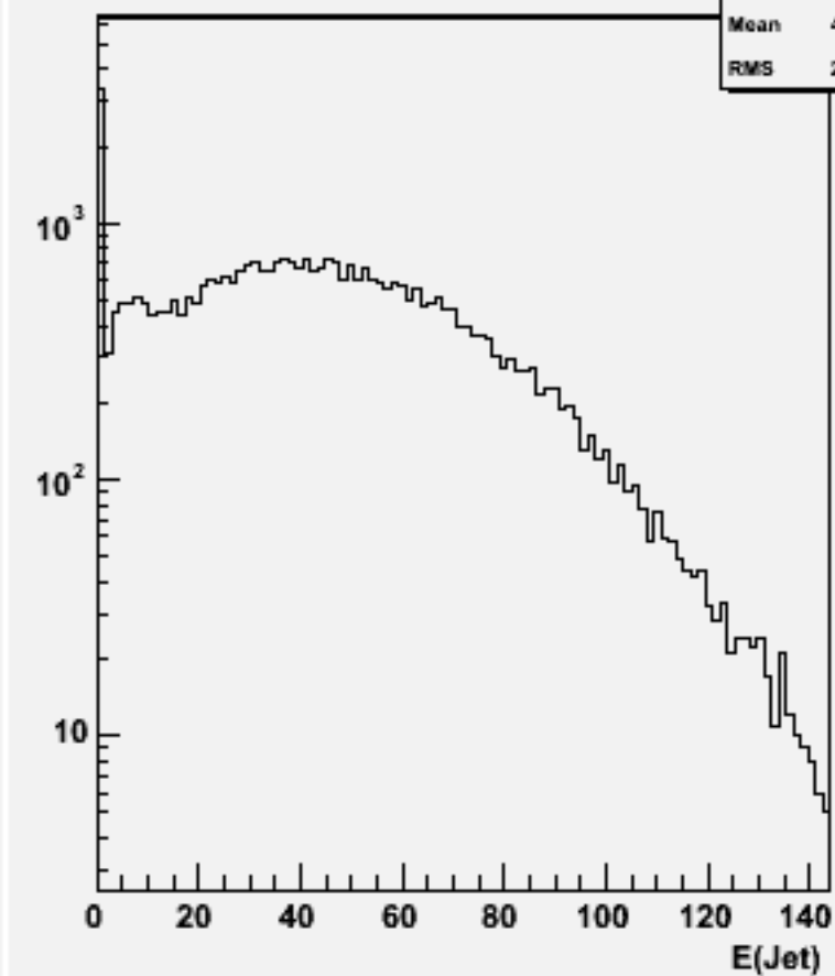
Jet energies(All jets)w101529 n3n3n2e2du_o
