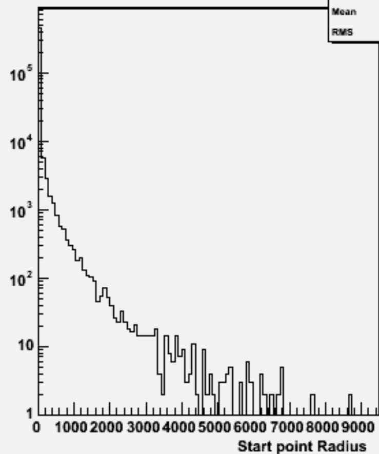
Start point R : w101528 n3n3n2e2du_o
