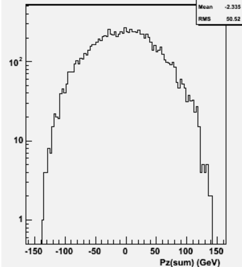
Pz Sum: w101528 n3n3n2e2du_o
