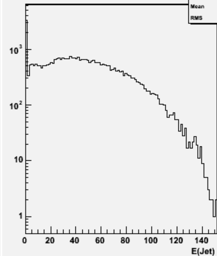
Jet energies(All jets)w101528 n3n3n2e2du_o
