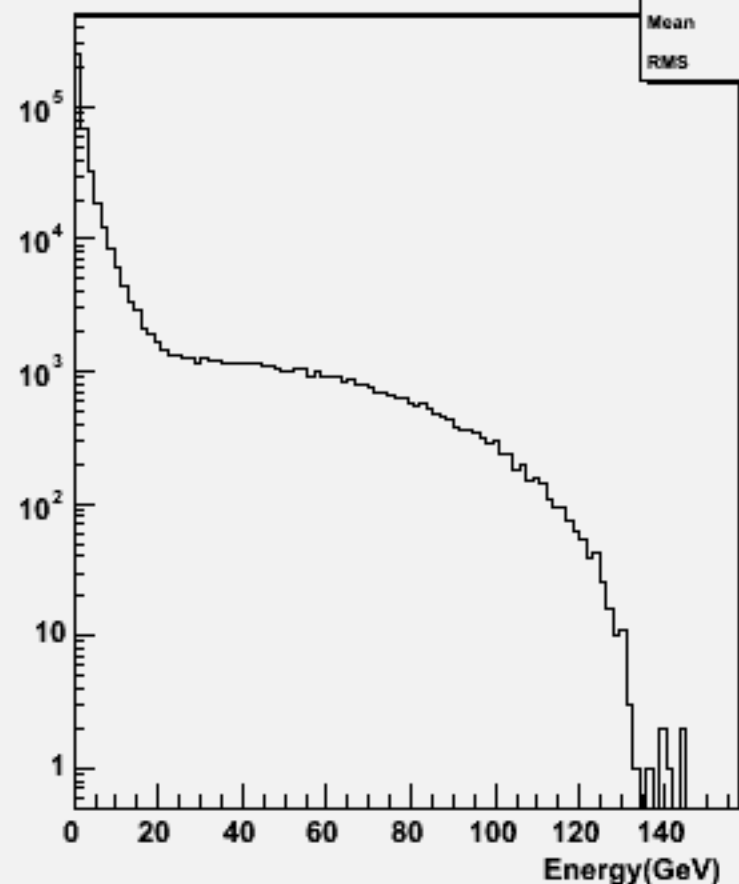
Start point R : w101528 n3n3n2e2du_o
