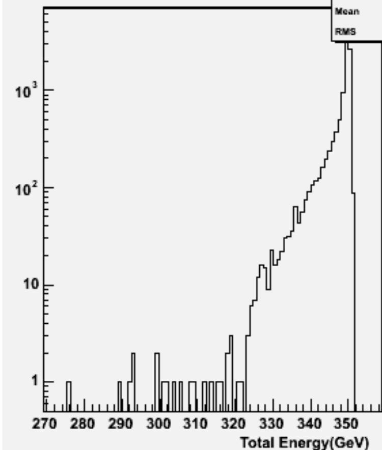
Pt Sum: w101528 n3n3n2e2du_o
