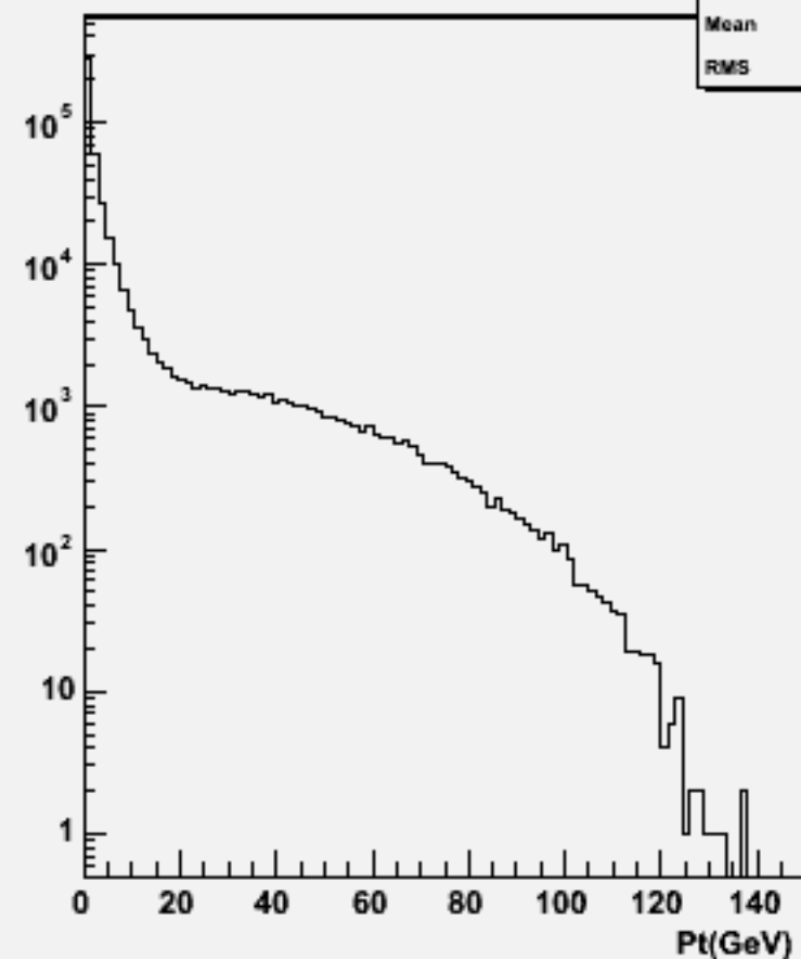
Start point Z : w101528 n3n3n2e2du_o
