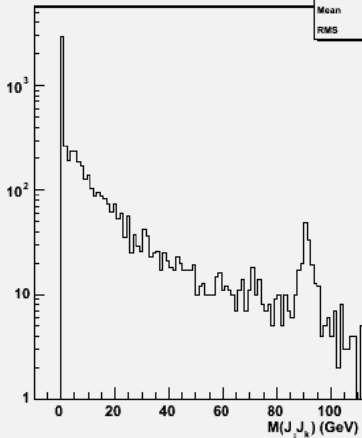
2jets mass(All comb)w101521 n3n3n2e2e2n2_o
