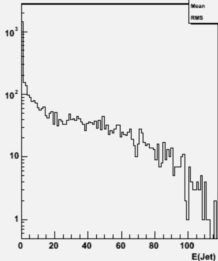
Jet energies(All jets)w101521 n3n3n2e2e2n2_o
