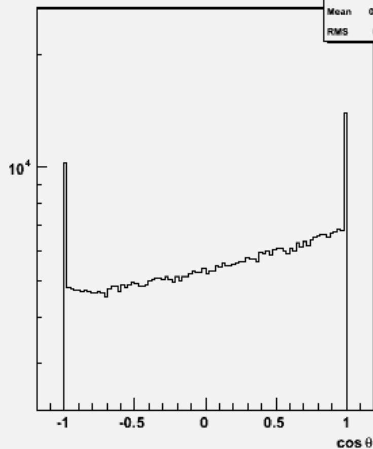
Particle cosθ : w101513 n3n3n1e1sc_o
