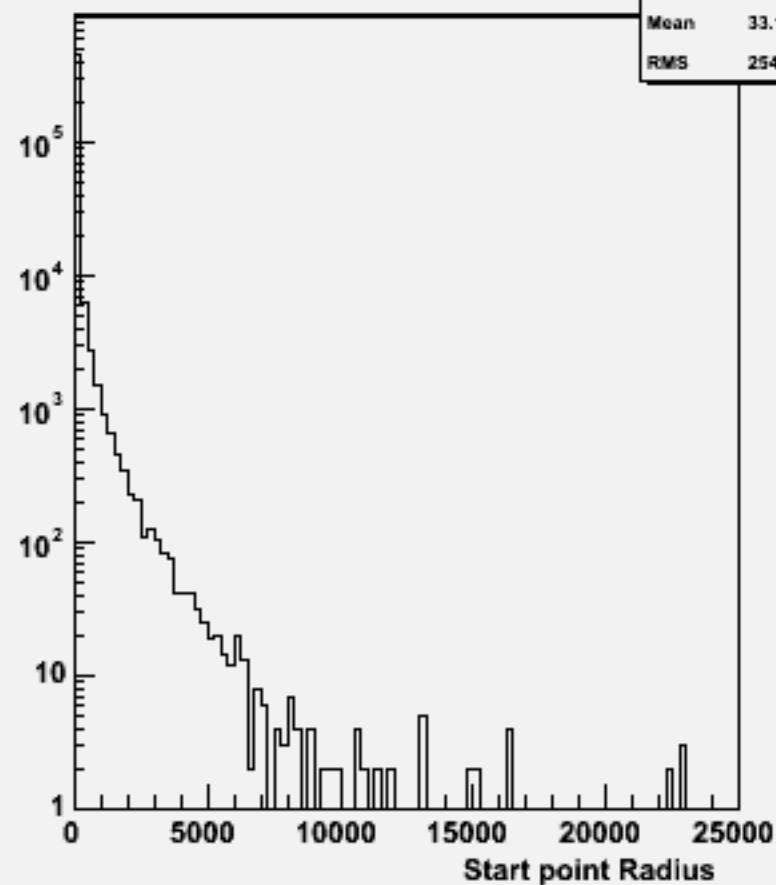
Start point R : w101513 n3n3n1e1sc_o
