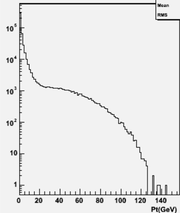
Particle Pt : w101513 n3n3n1e1sc_o
