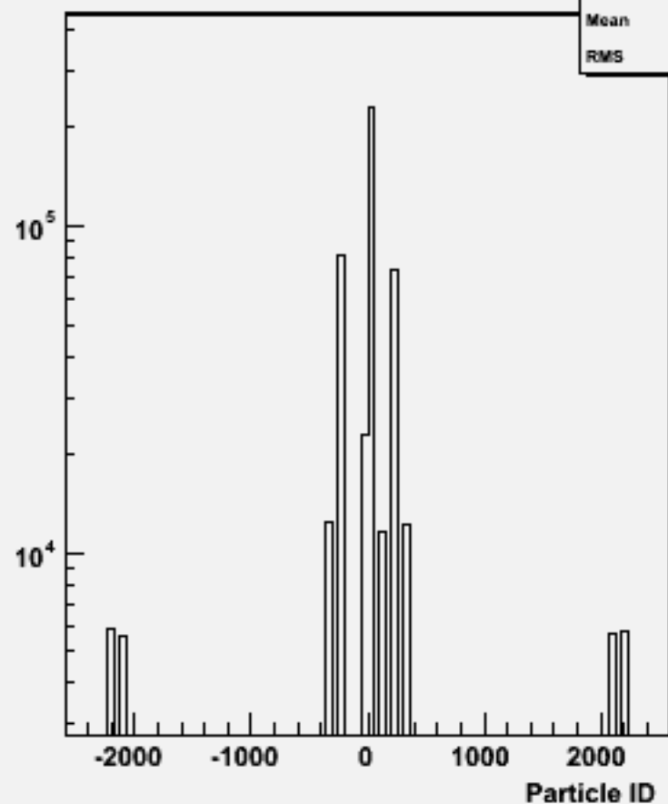
Particle ID : w101513 n3n3n1e1sc_o
