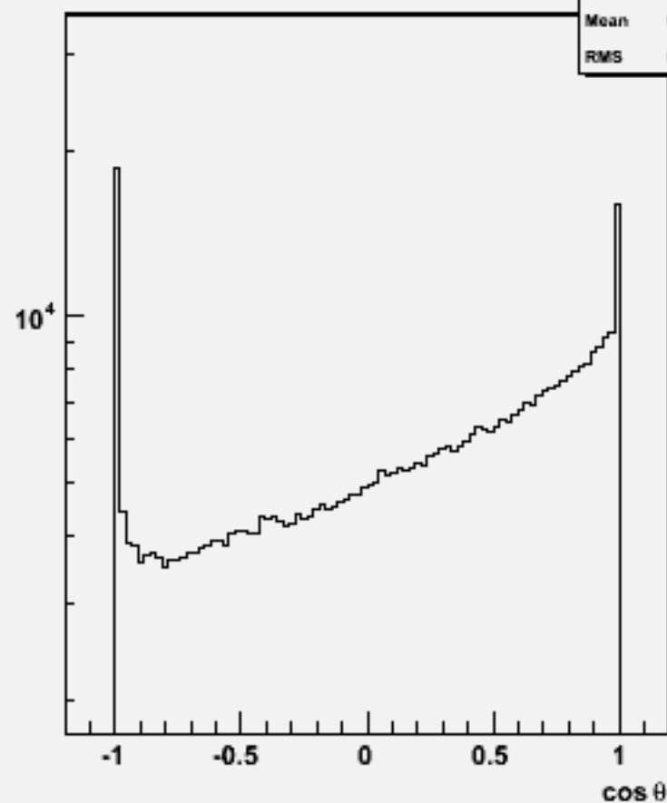
Particle \cos\theta : w101511 n3n3n1e1sc_o
