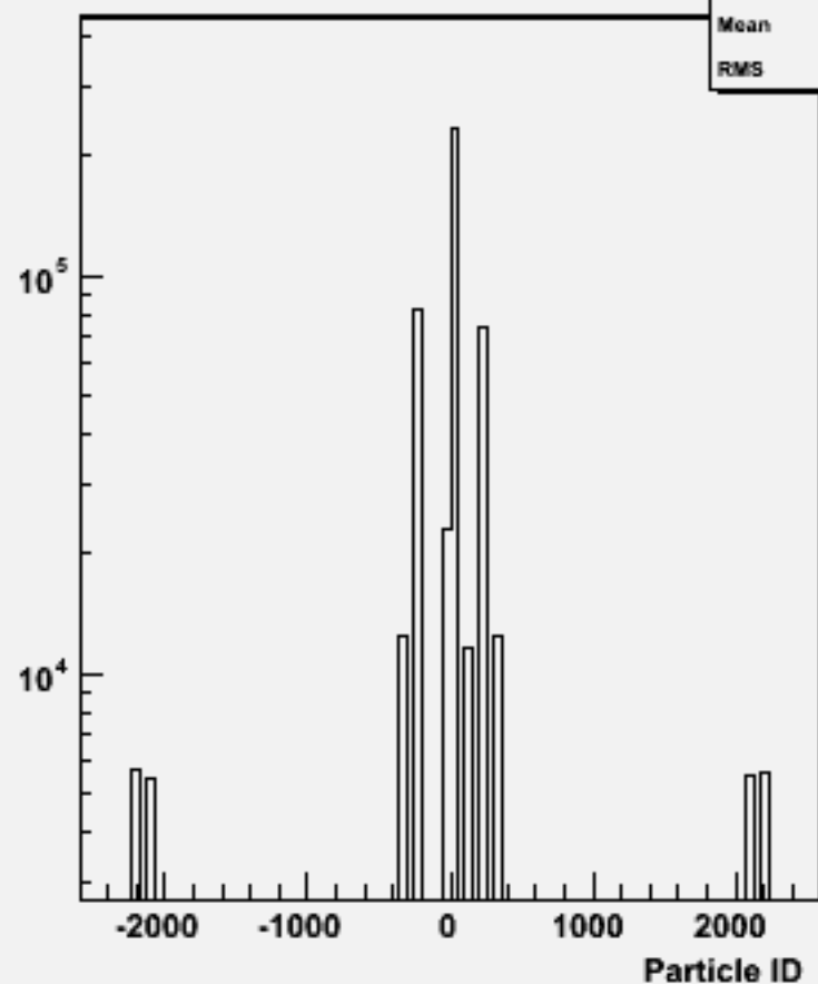
Particle ID : w101511 n3n3n1e1sc_o
