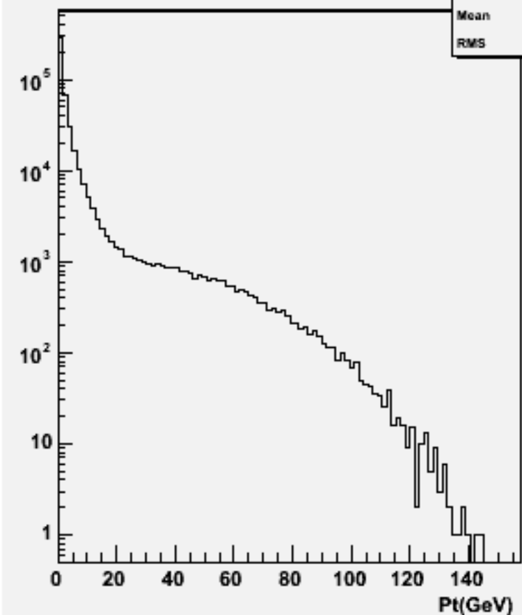
Particle Pt : w101511 n3n3n1e1sc_o
