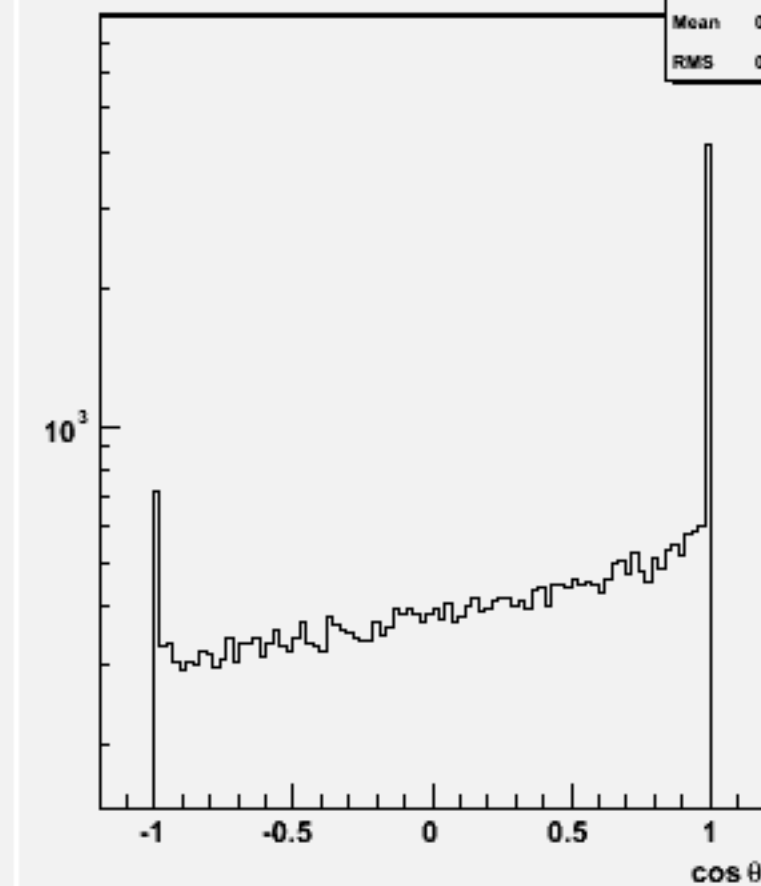
Jet cos \theta (All jets)w101509 n3n3n1e1du_o
