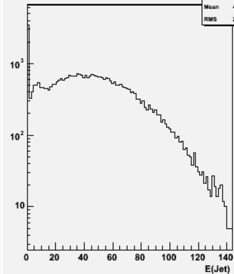
Jet energies(All jets)w101509 n3n3n1e1du_o
