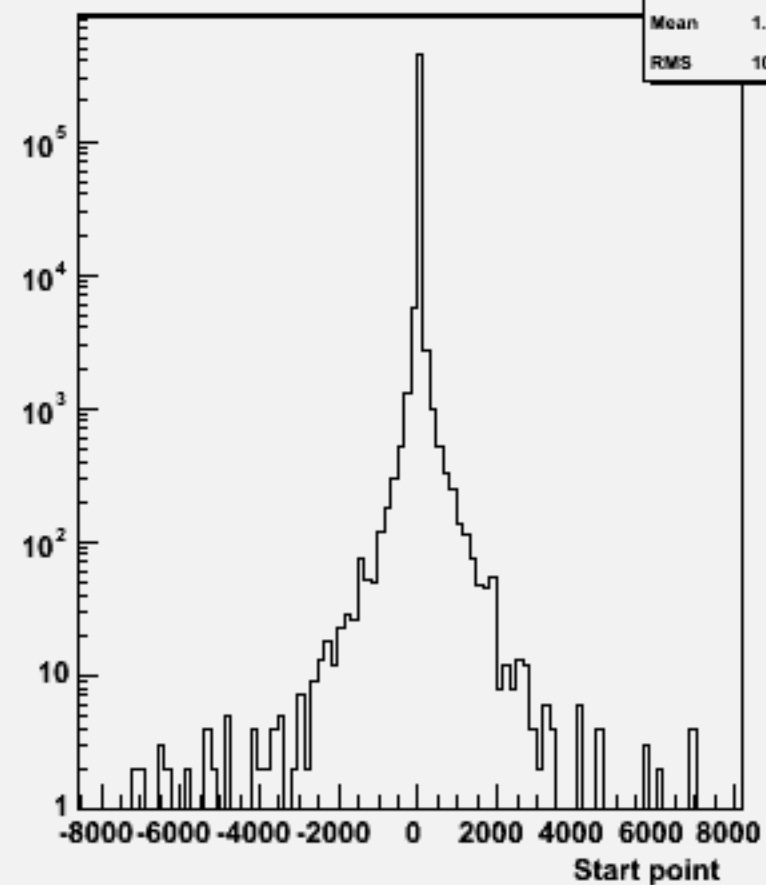
Start point Z : w101509 n3n3n1e1du_o
