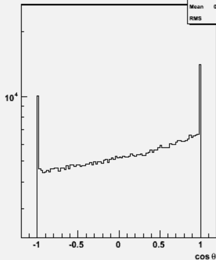
Particle cosθ : w101509 n3n3n1e1du_o
