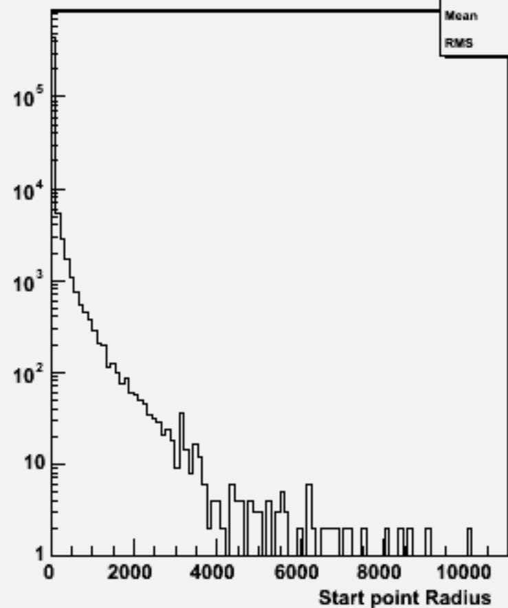
Start point R : w101509 n3n3n1e1du_o
