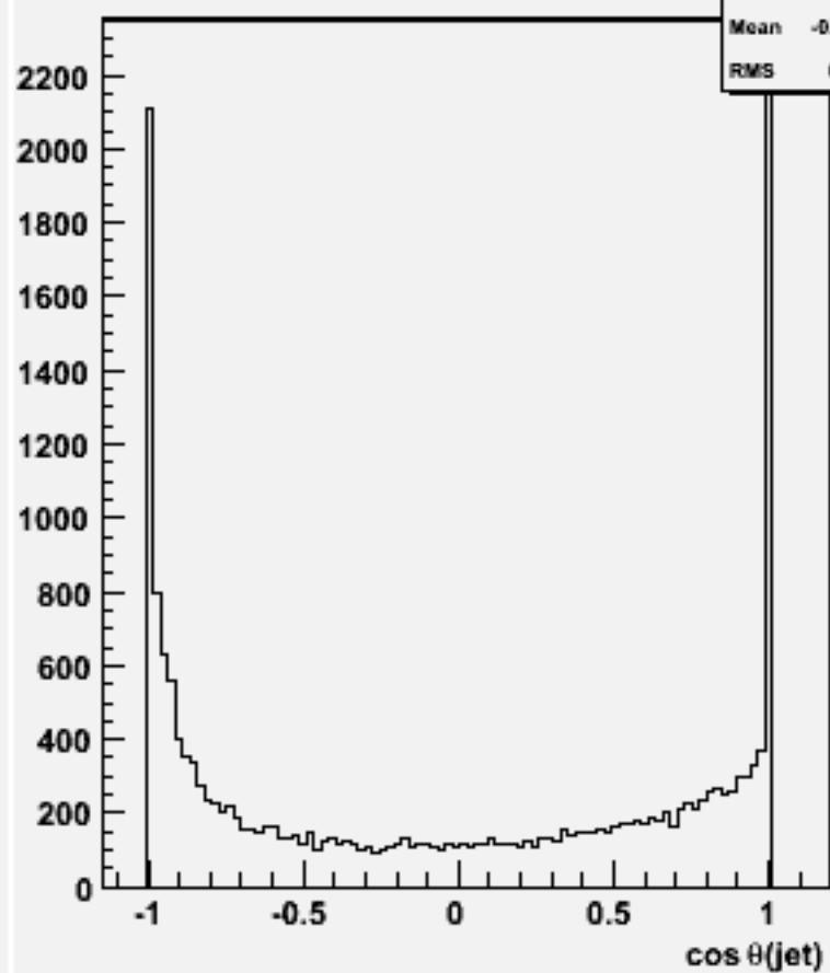
cos \theta for 2-jets :w101508 n3n3n1e1du_o
