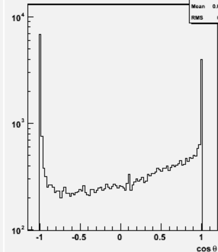
Jet cos \theta (All jets)w101508 n3n3n1e1du_o
