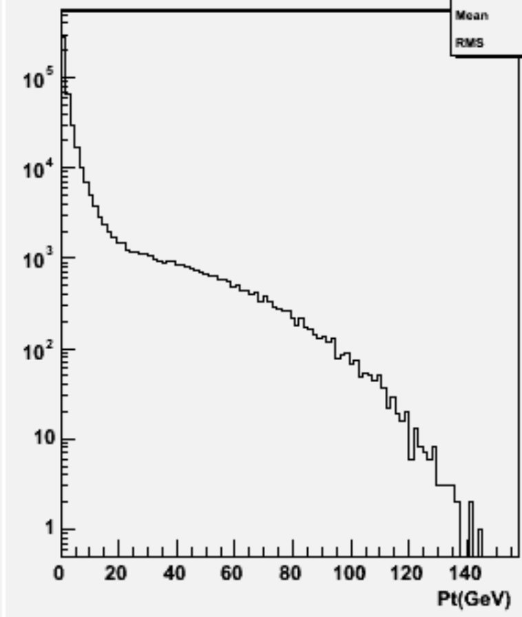
Start point Z : w101507 n3n3n1e1du_o
