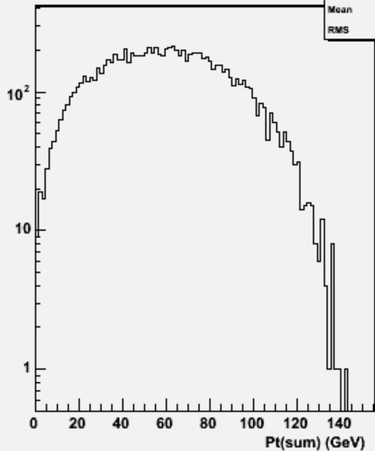
Pt Sum: w101507 n3n3n1e1du_o
