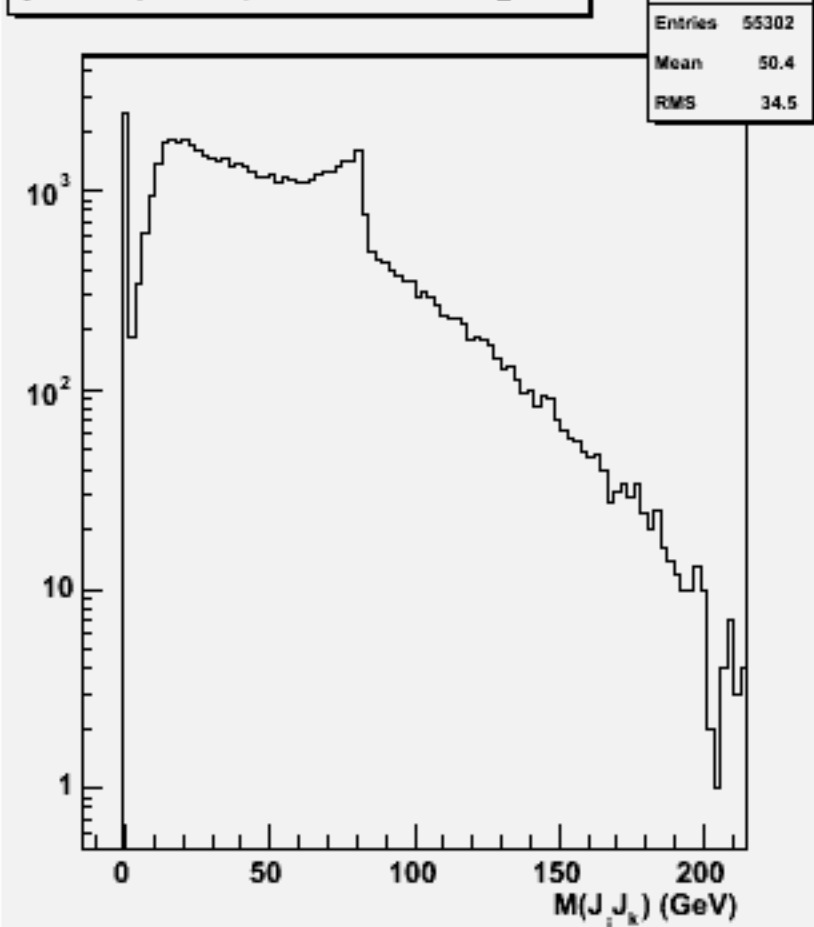
2jets mass(All comb)w101507 n3n3n1e1du_o
