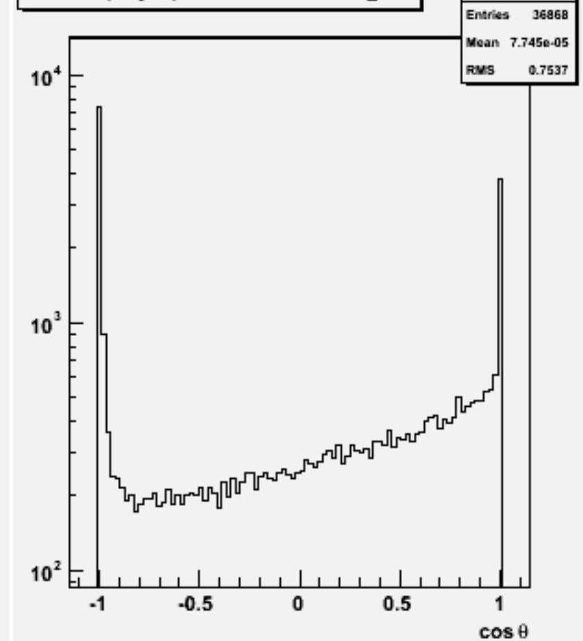
Jet cos \theta (All jets)w101507 n3n3n1e1du_o
