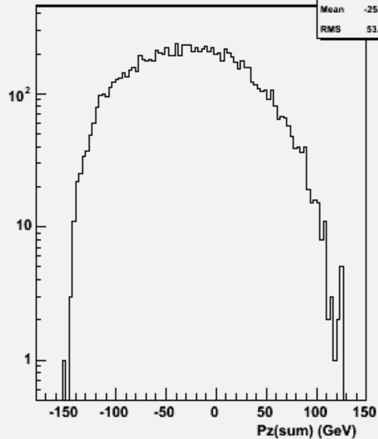
Pz Sum: w101507 n3n3n1e1du_o
