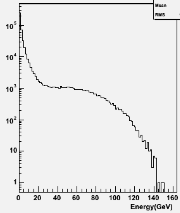
Start point R : w101507 n3n3n1e1du_o
