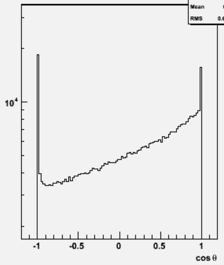
Particle cosθ : w101507 n3n3n1e1du_o
