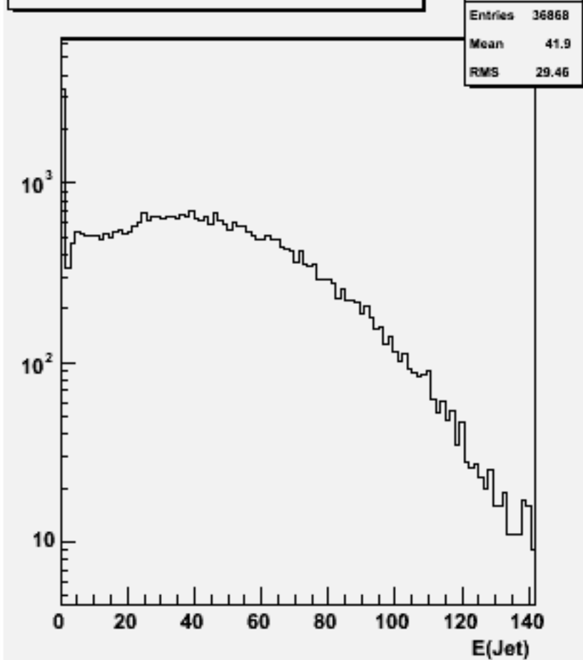
Jet energies(All jets)w101507 n3n3n1e1du_o
