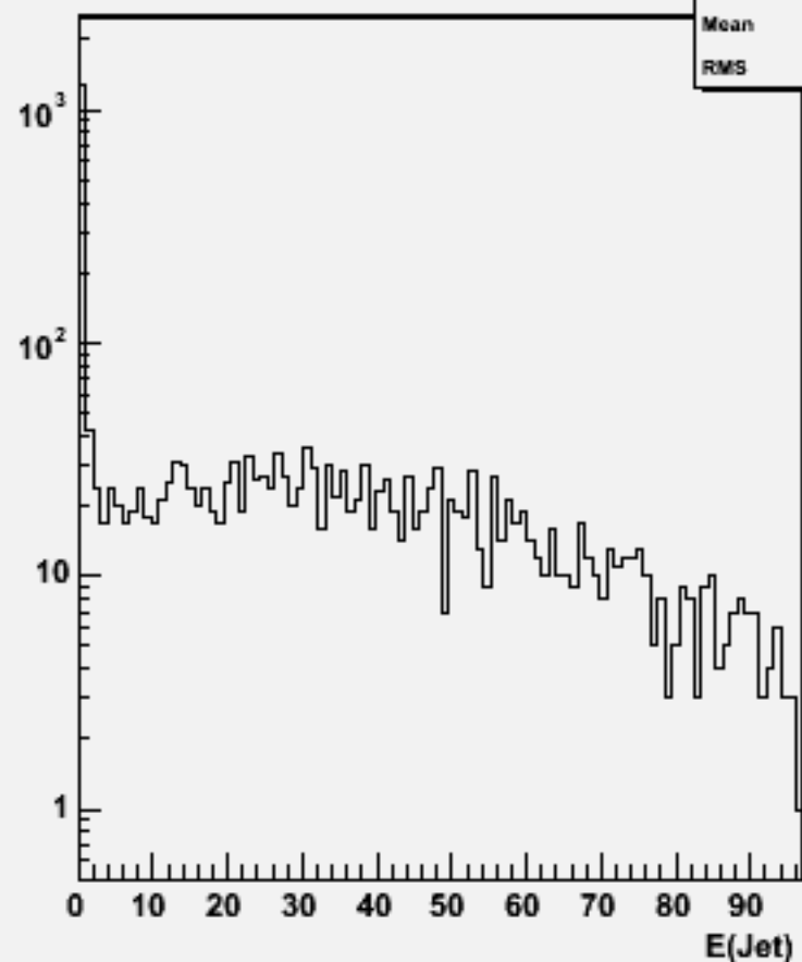
Jet energies(All jets)w101504 n3n3n1e1e3n3_o
