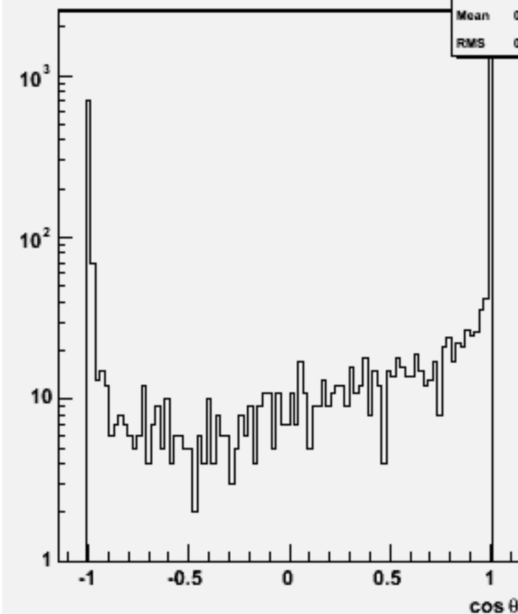
Jet cos \theta (All jets)w101503 n3n3n1e1e3n3_o
