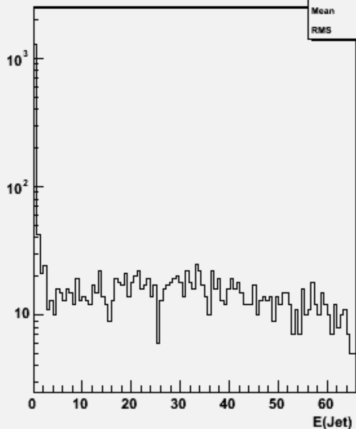
Jet energies(All jets)w101503 n3n3n1e1e3n3_o
