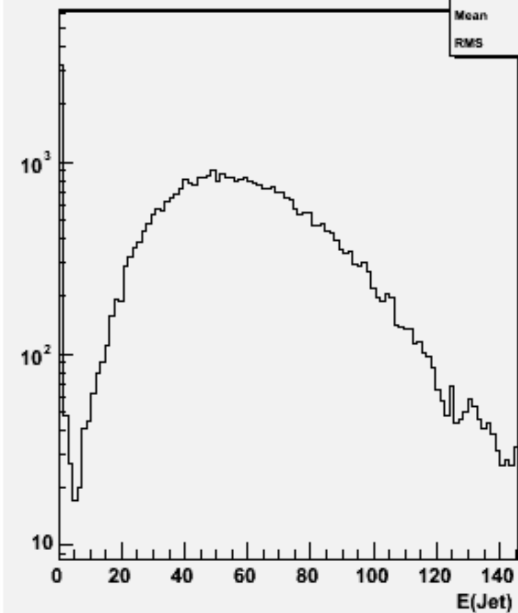
Jet energies(All jets)w101473 n2n2udsc_o
