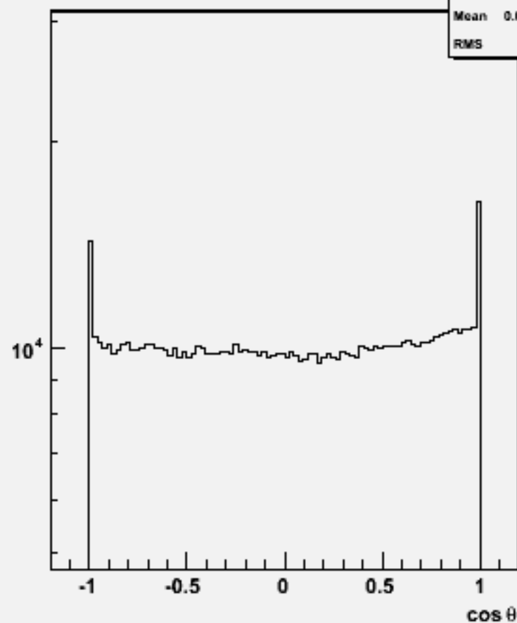
Particle cos \theta : w101473 n2n2udsc_o
