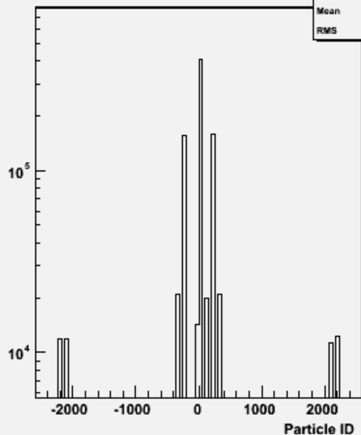
Particle ID : w101473 n2n2udsc_o
