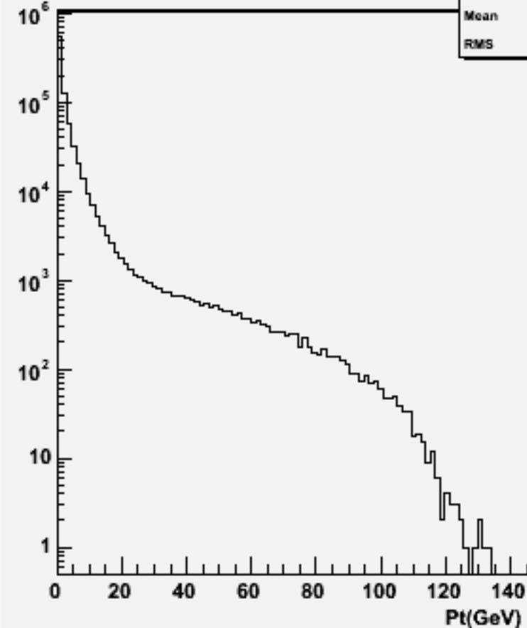
Particle Pt : w101473 n2n2udsc_o
