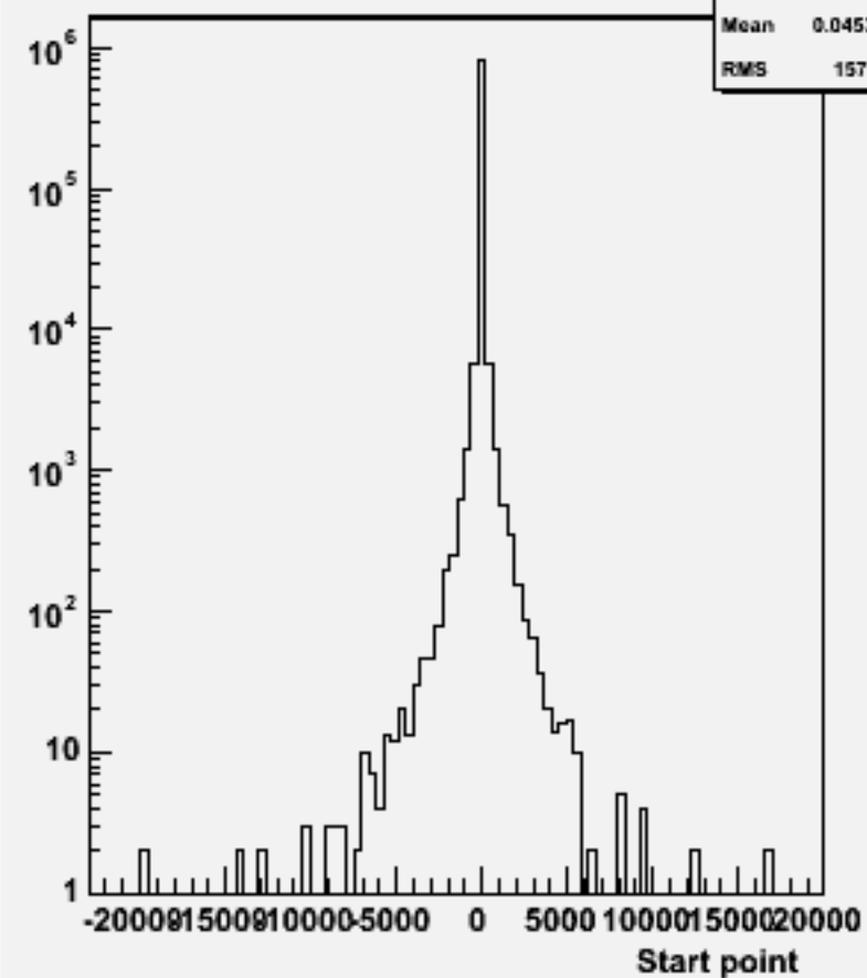
Start point Z : w101473 n2n2udsc_o
