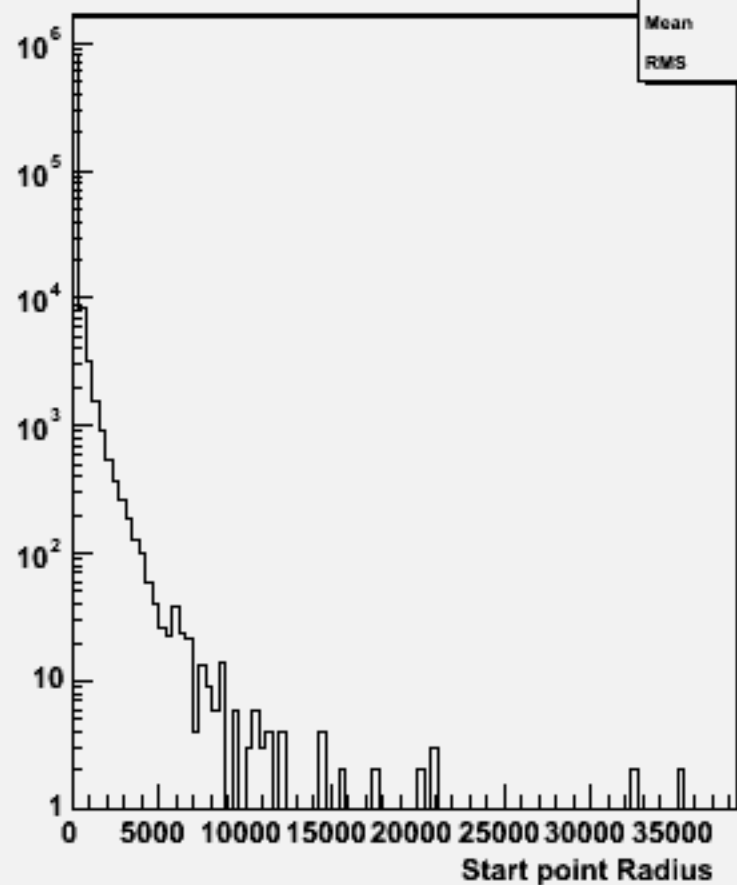
Start point R : w101473 n2n2udsc_o
