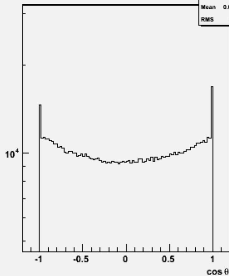
Particle cos \theta : w101472 n2n2udsc_o
