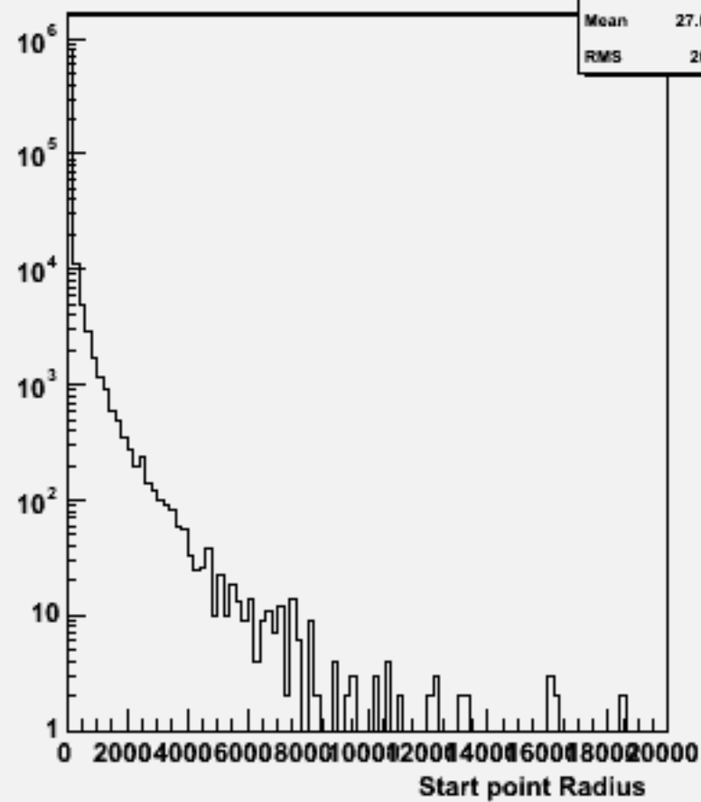
Start point R : w101472 n2n2udsc_o
