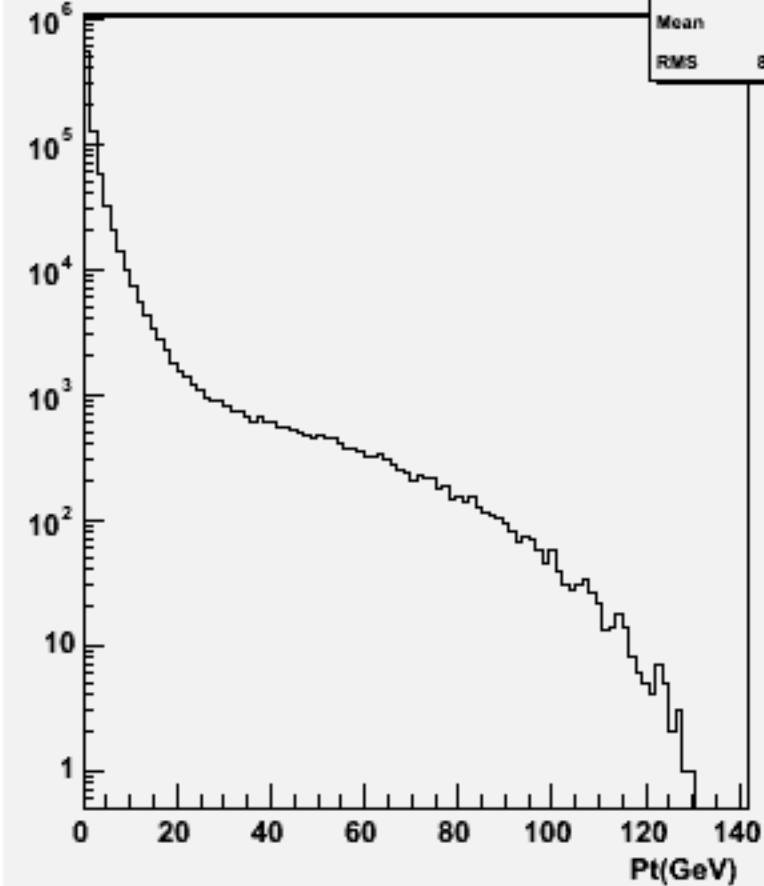
Particle Pt : w101472 n2n2udsc_o
