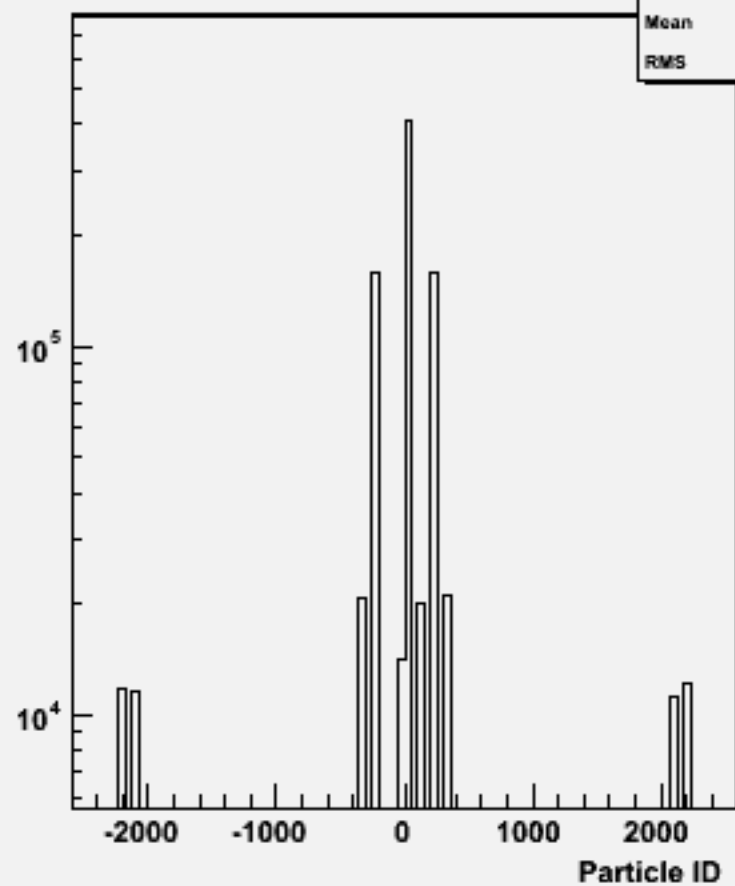
Particle ID : w101472 n2n2udsc_o
