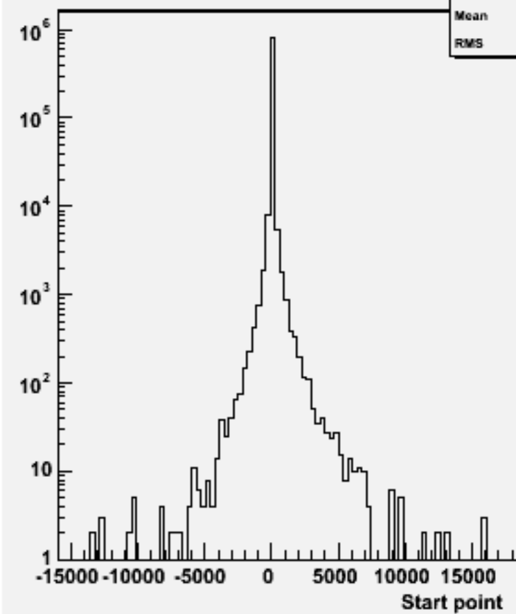
Start point Z : w101472 n2n2udsc_o
