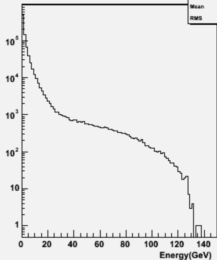
Particle Energy : w101472 n2n2udsc_o
