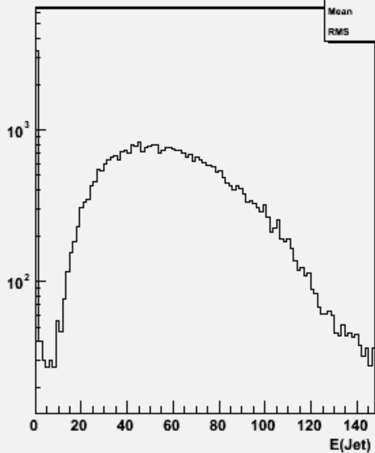
Jet energies(All jets)w101472 n2n2udsc_o
