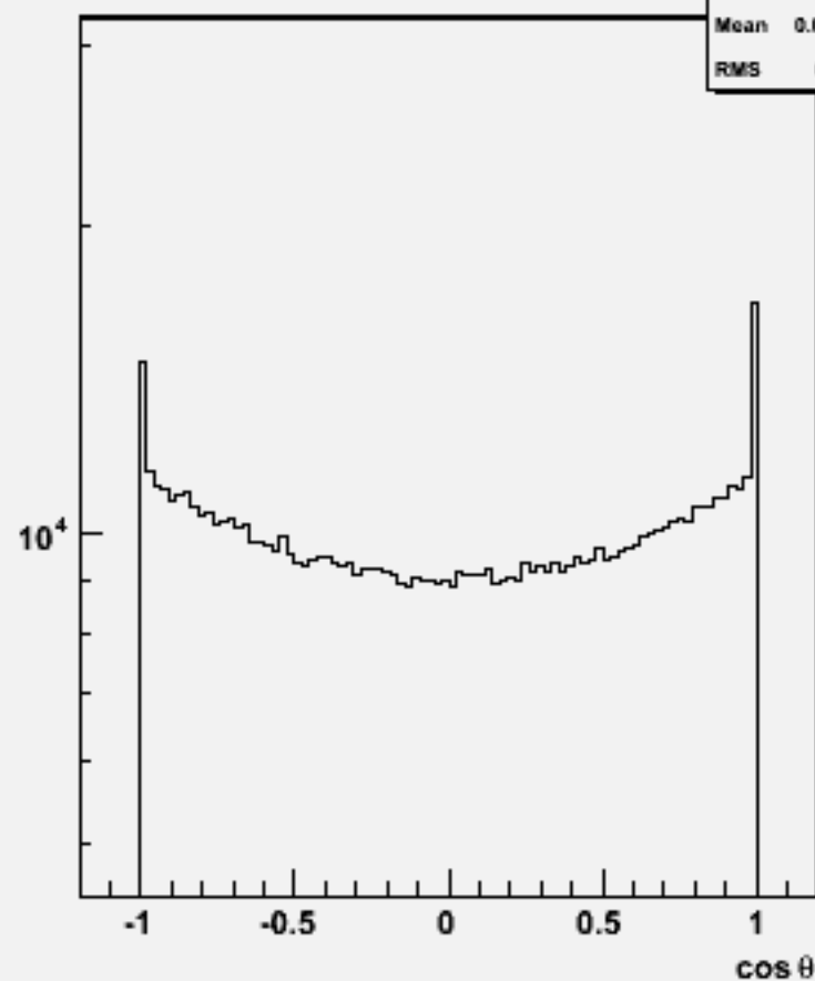
Particle cos \theta : w101468 n2n2uddu_o
