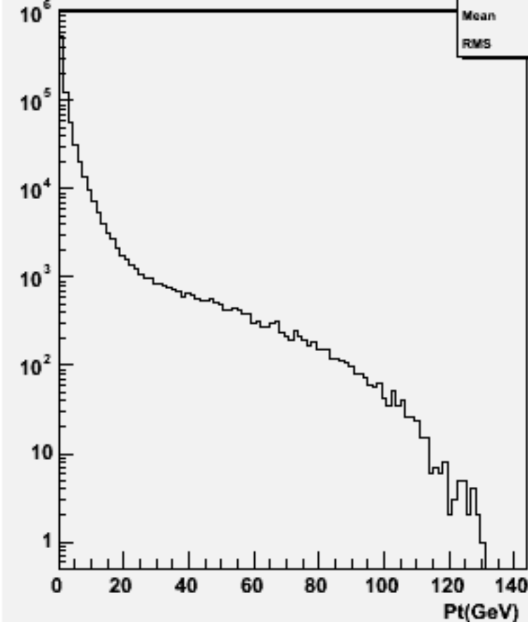
Particle Pt : w101468 n2n2uddu_o
