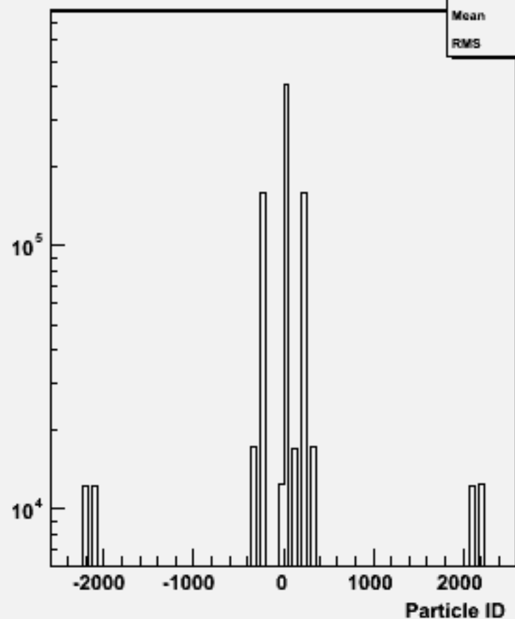
Particle ID : w101468 n2n2uddu_o
