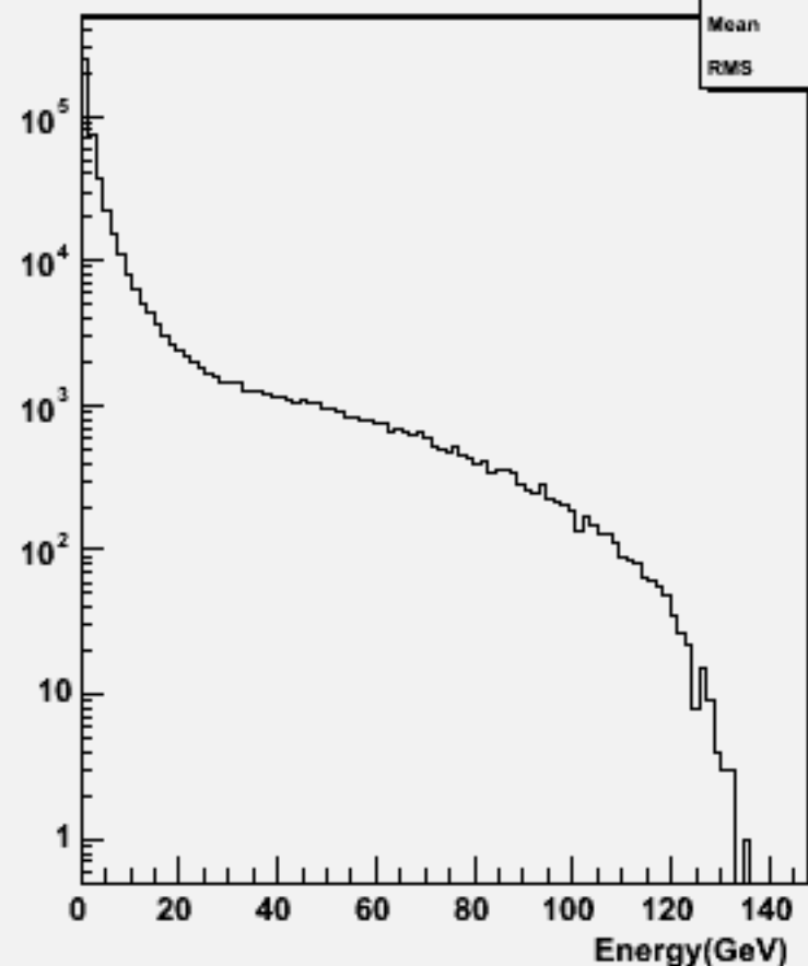
Start point R : w101464 n2n2ude3n3_o
