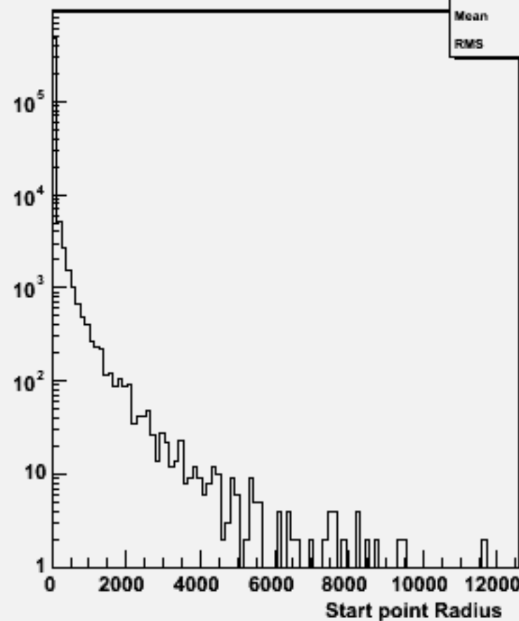
Start point R : w101464 n2n2ude3n3_o
