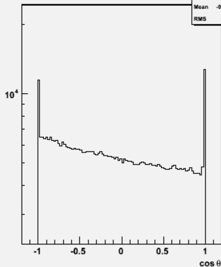
Particle cos \theta : w101461 n2n2ude2n2_o
