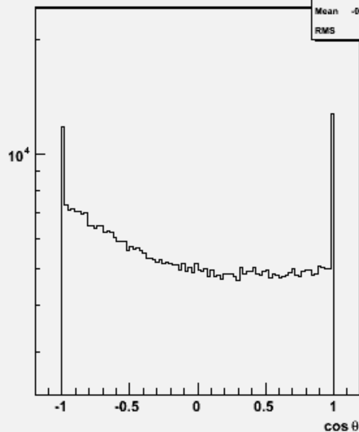
Particle cos \theta : w101460 n2n2ude2n2_o
