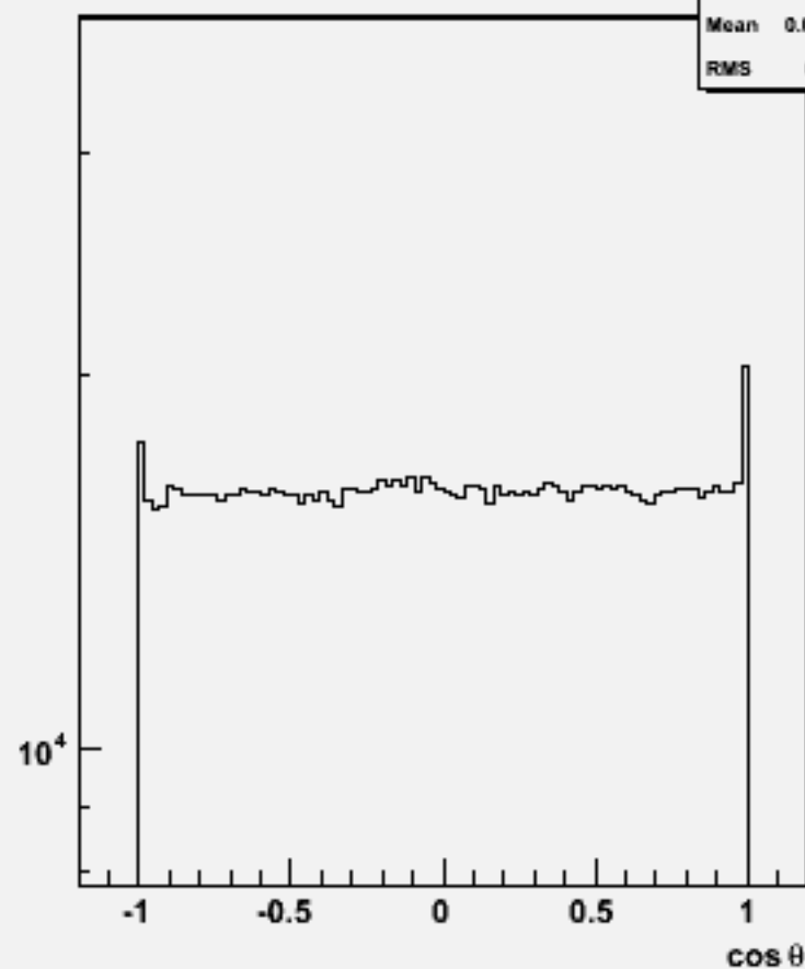
Particle cosθ : w101273 bbudsc_o
