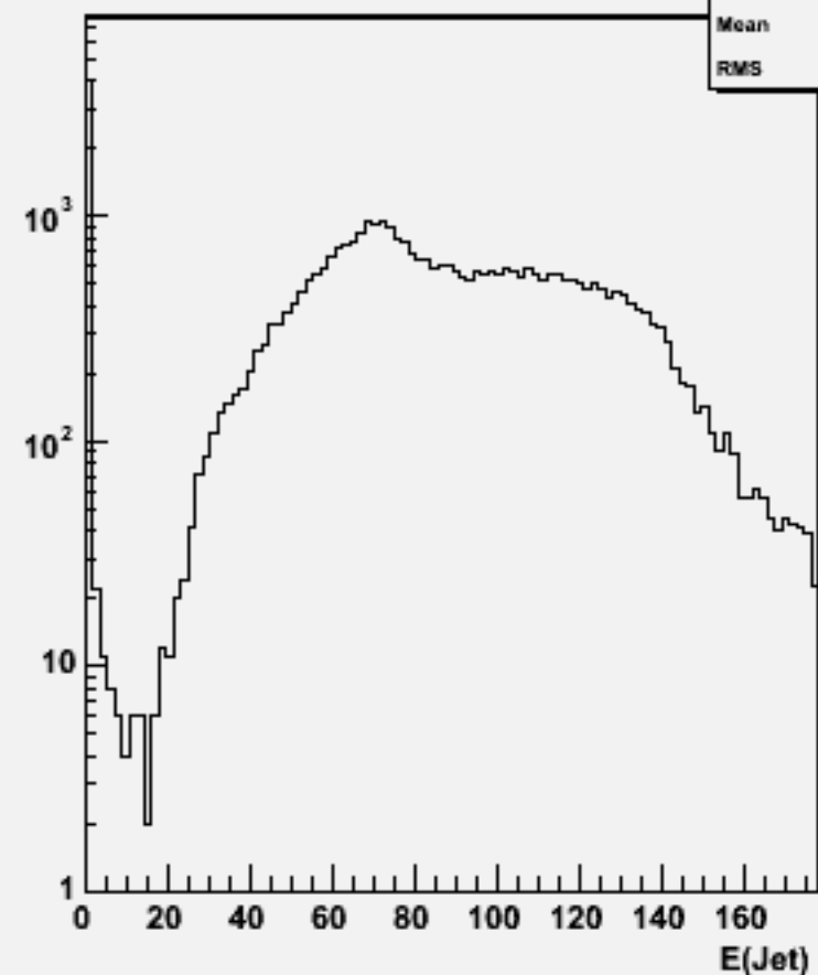
Jet energies(All jets)w101273 bbudsc_o
