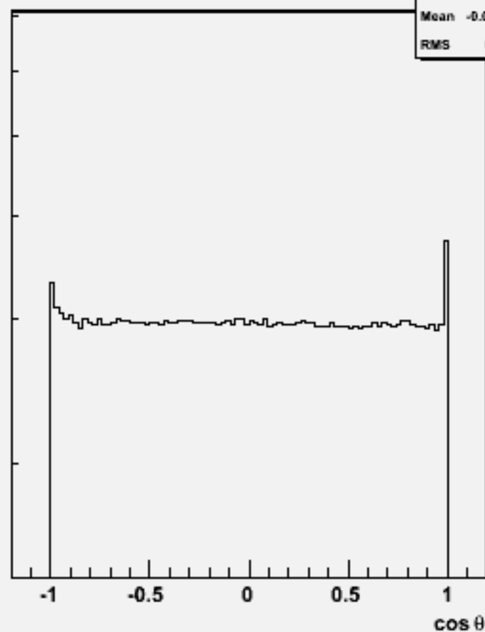
Particle \cos\theta : w101272 bbudsc_o
