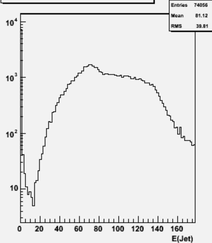
Jet energies(All jets)w101272 bbudsc_o
