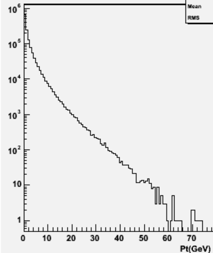
Particle Pt : w101269 bbuddu_o
