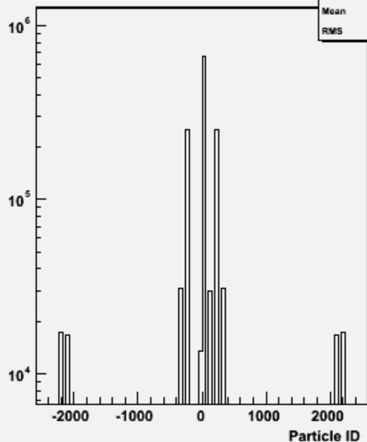
Particle ID : w101269 bbuddu_o
