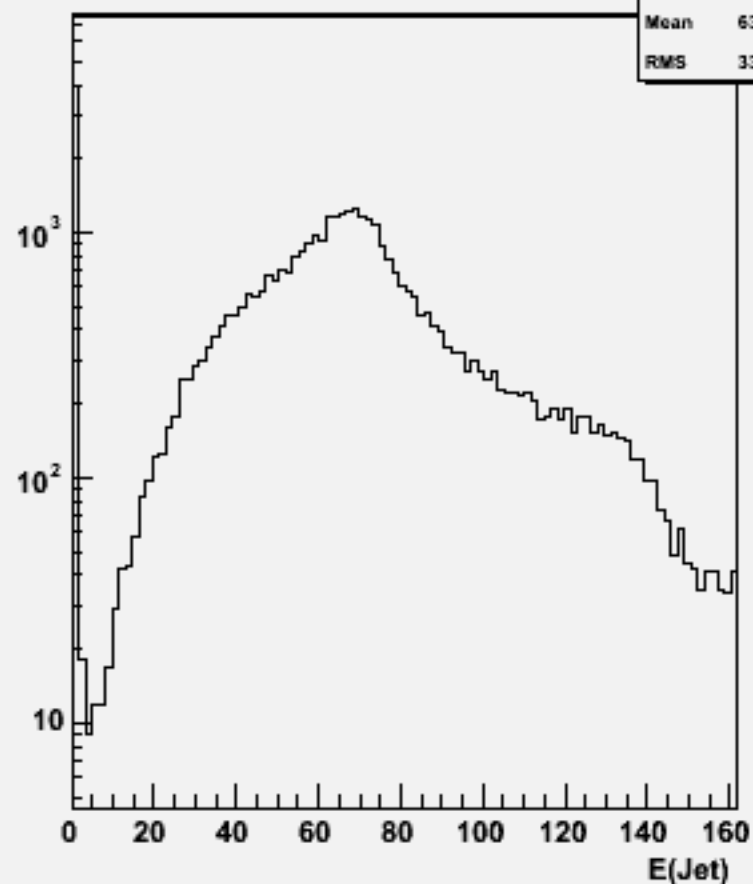
Jet energies(All jets)w101265 bbude3n3_o
