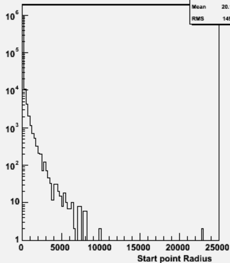
Start point R : w101265 bbude3n3_o
