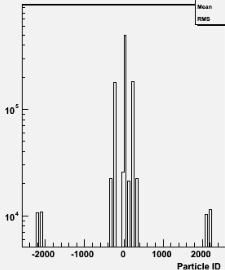
Particle ID : w101265 bbude3n3_o
