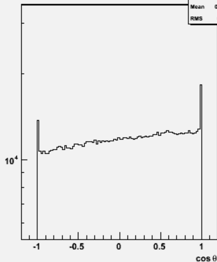
Particle cos \theta : w101265 bbude3n3_o
