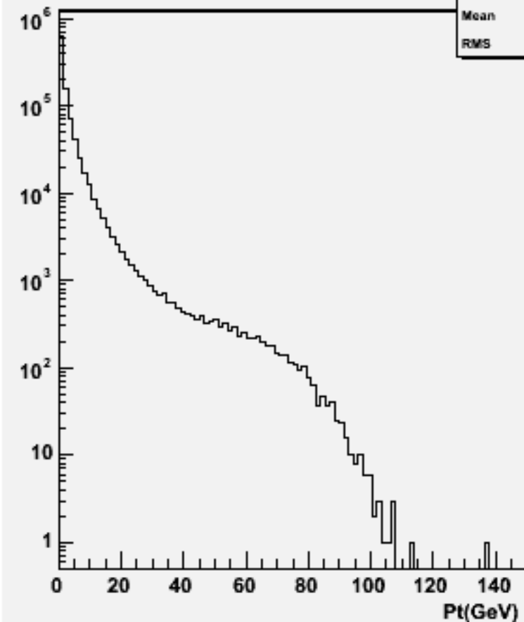
Particle Pt : w101265 bbude3n3_o
