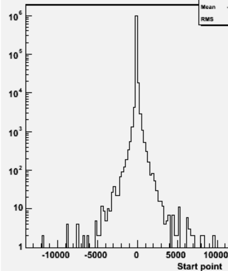
Start point Z : w101264 bbude3n3_o
