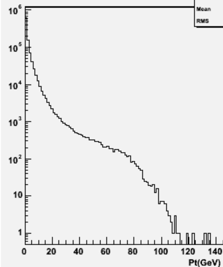
Particle Pt : w101264 bbude3n3_o
