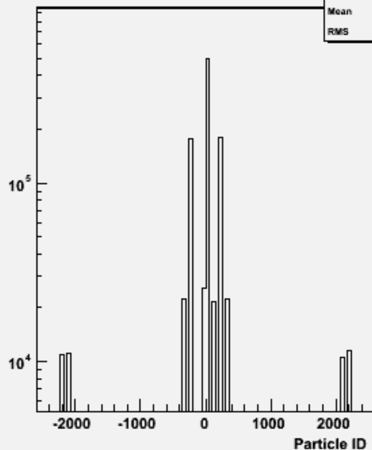
Particle ID : w101264 bbude3n3_o
