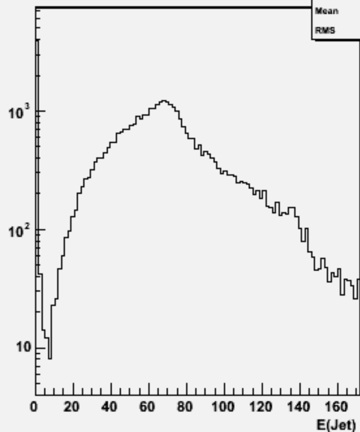
Jet energies(All jets)w101264 bbude3n3_o
