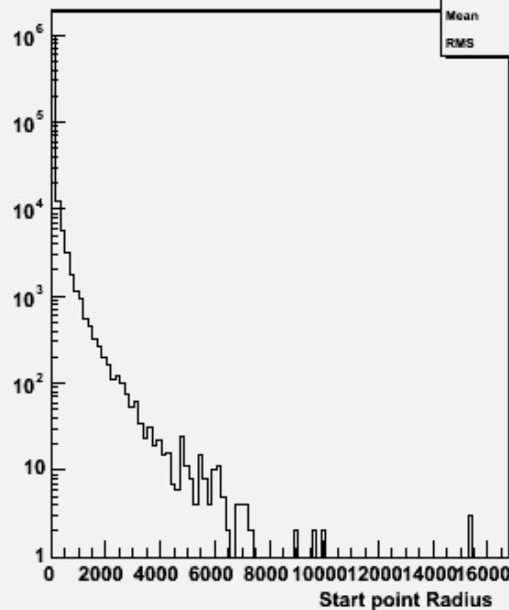
Start point R : w101264 bbude3n3_o
