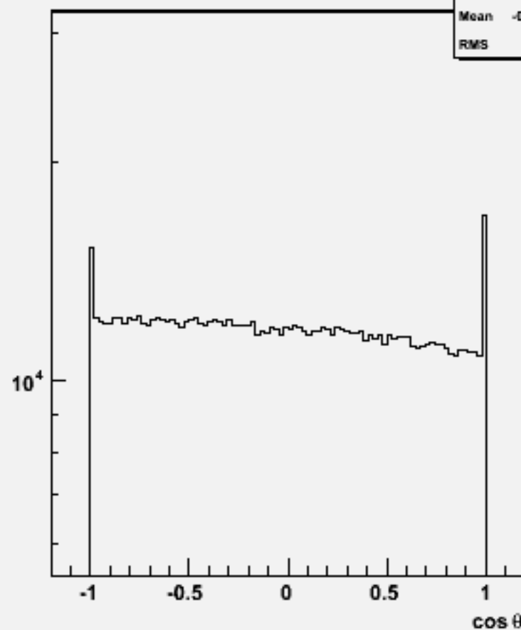
Particle cos \theta : w101264 bbude3n3_o
