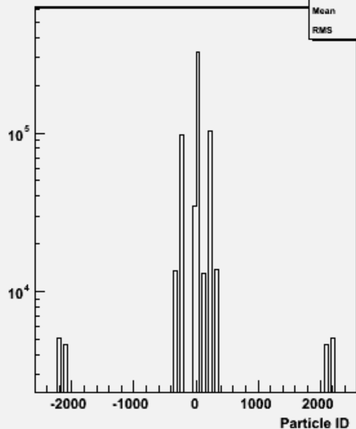
Particle ID : w101241 bbn3e3e2n2_o
