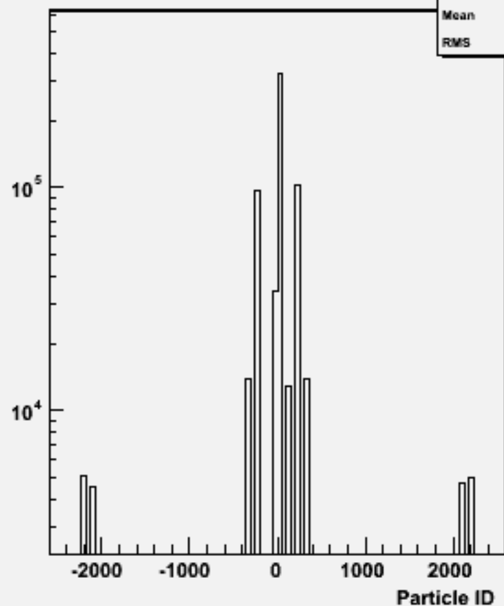
Particle ID : w101240 bbn3e3e2n2_o
