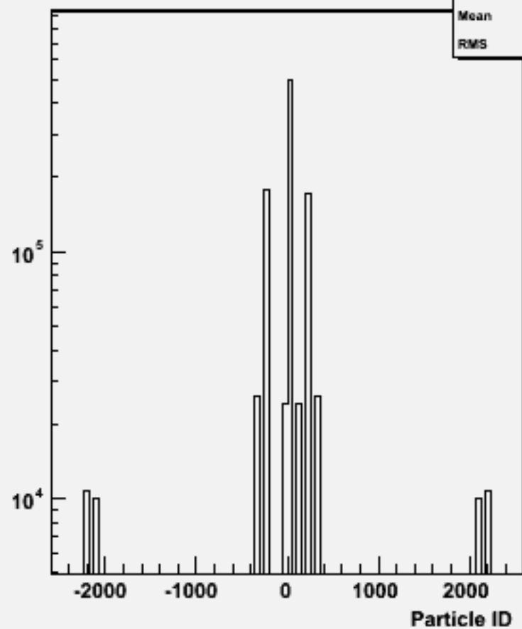
Particle ID : w101233 bbn2e2sc_o
