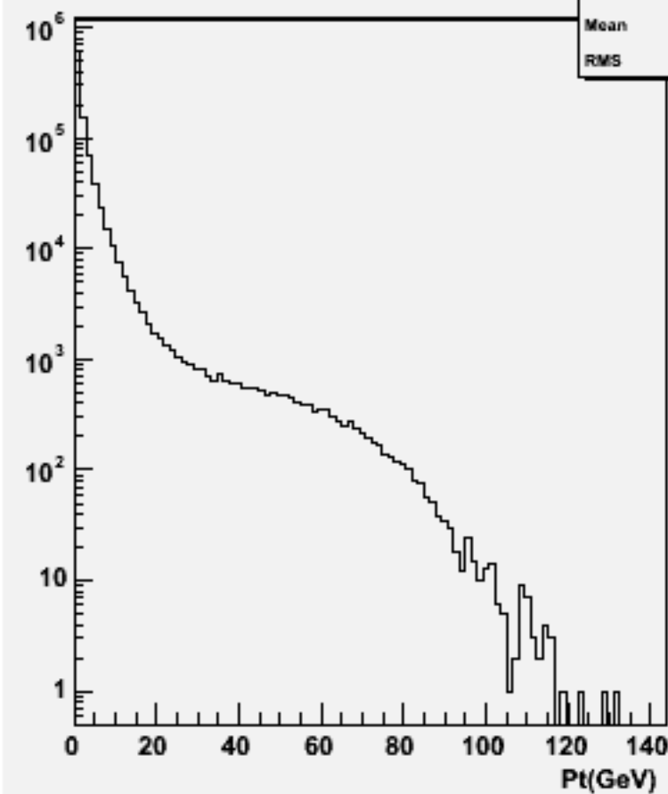
Particle Pt : w101228 bbn2e2du_o
