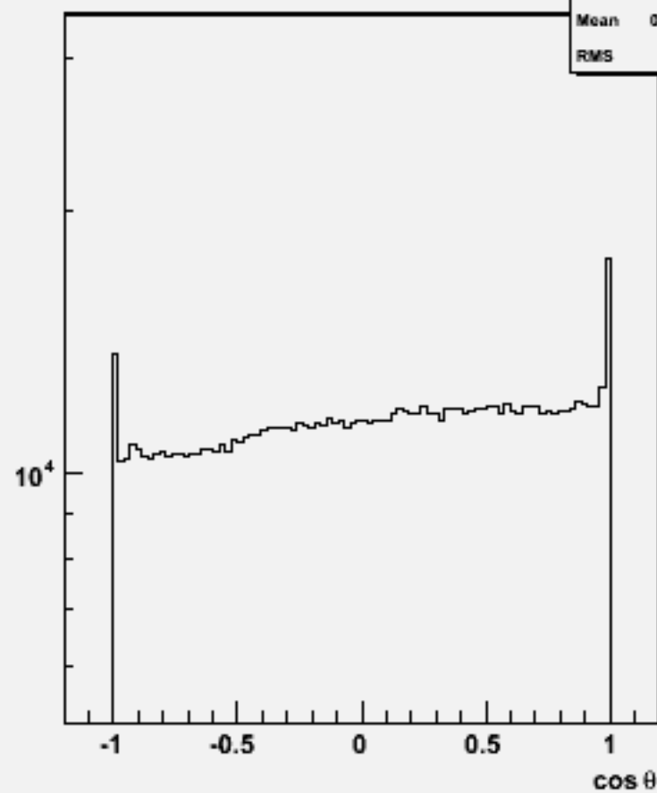
Particle cos \theta : w101228 bbn2e2du_o
