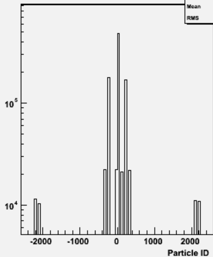
Particle ID : w101228 bbn2e2du_o
