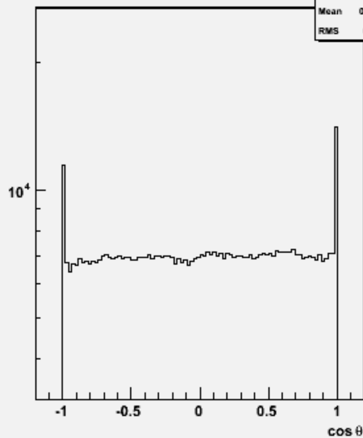
Particle cosθ : w101220 bbn2e2e2n2_o
