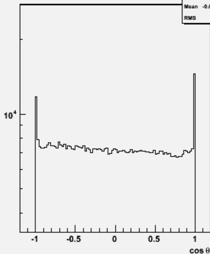
Particle cos \theta : w101205 bbn1e1e3n3_o
