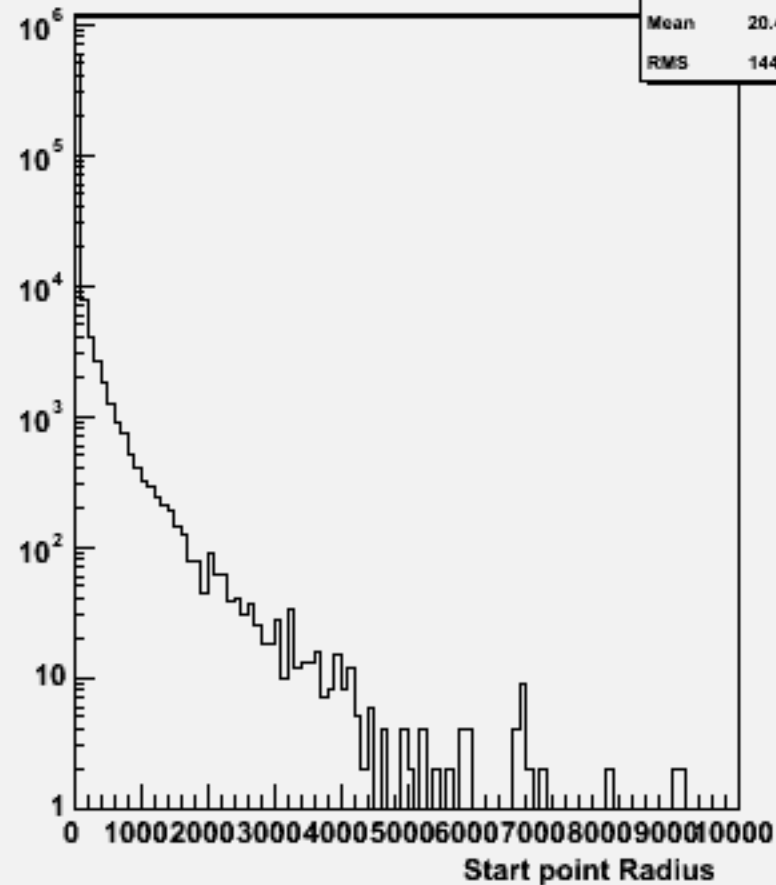
Start point R : w101205 bbn1e1e3n3_o
