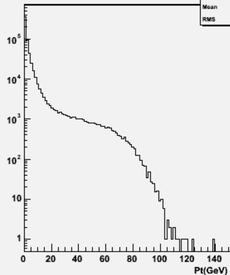
Particle Pt : w101205 bbn1e1e3n3_o
