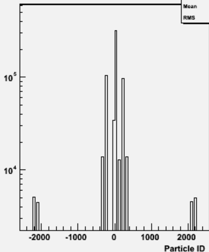
Particle ID : w101205 bbn1e1e3n3_o
