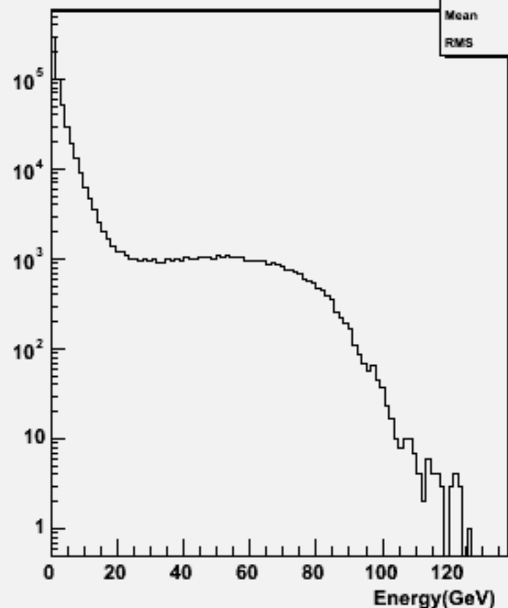
Start point R : w101201 bbn1e1e2n2_o
