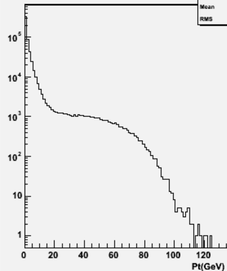
Start point Z : w101201 bbn1e1e2n2_o
