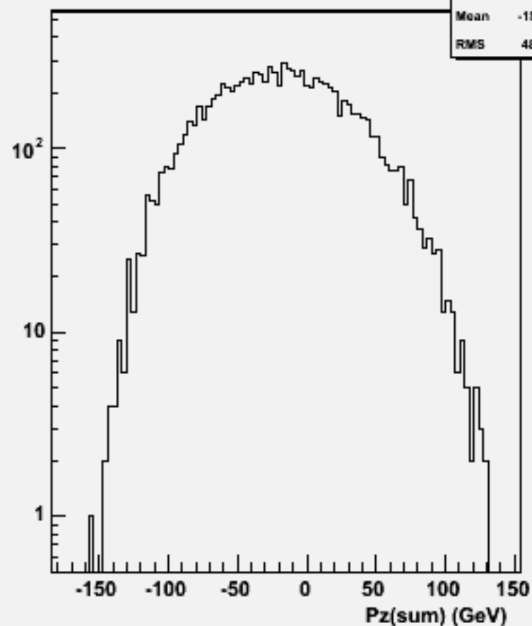
Pz Sum: w101200 bbn1e1e2n2_o
