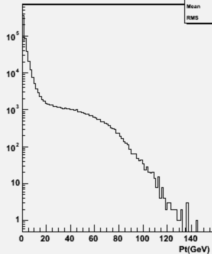
Start point Z : w101200 bbn1e1e2n2_o
