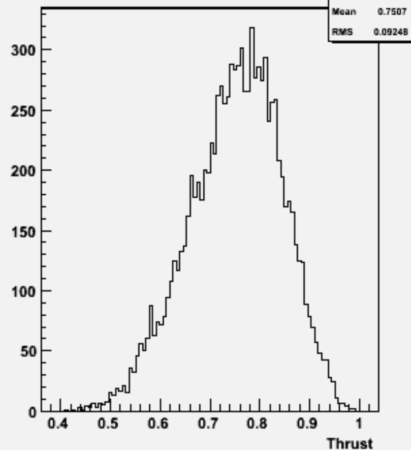
Thrust w101200 bbn1e1e2n2_o
