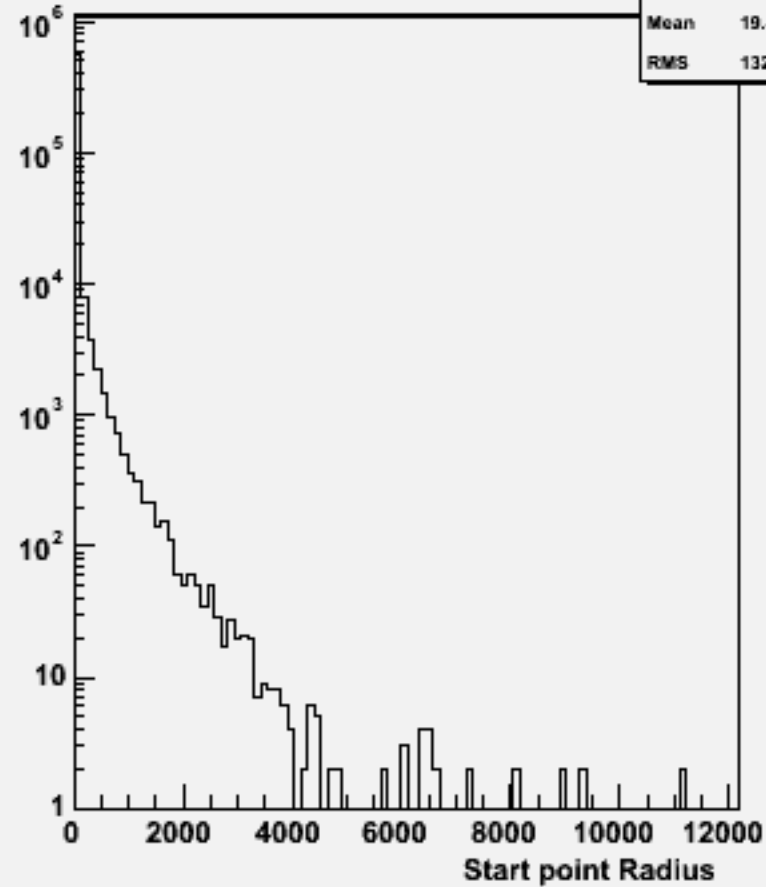
Start point R : w101200 bbn1e1e2n2_o
