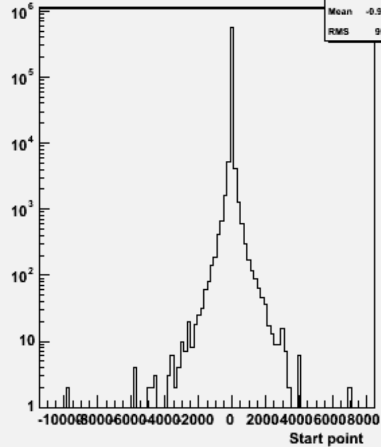
Start point Z : w101200 bbn1e1e2n2_o
