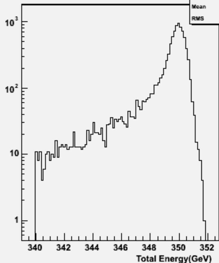
Pz Sum: w101200 bbn1e1e2n2_o
