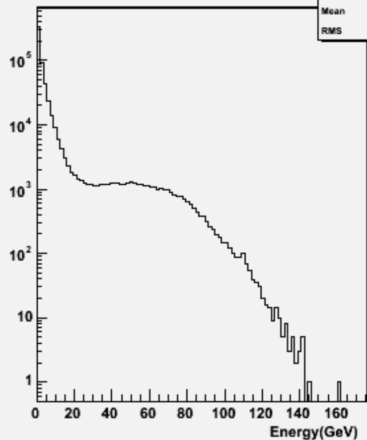
Start point R : w101200 bbn1e1e2n2_o
