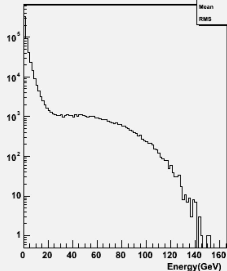
Start point R : w101199 bbn1e1e2n2_o
