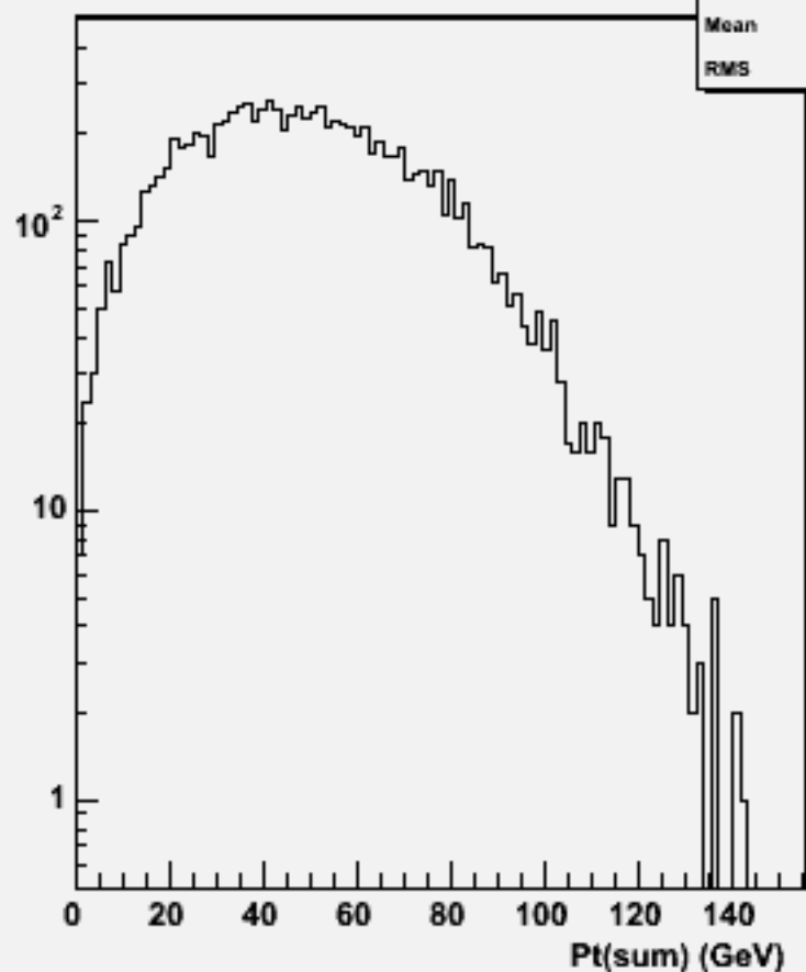
Pt Sum: w101199 bbn1e1e2n2_o
