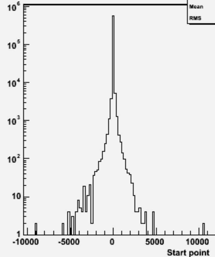
Start point Z : w101199 bbn1e1e2n2_o
