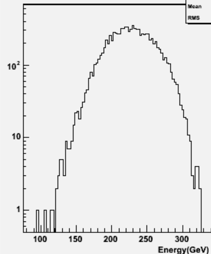
Thrust w101199 bbn1e1e2n2_o
