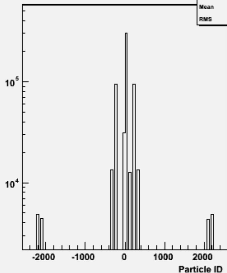
Particle ID : w101198 bbn1e1e1n1_o
