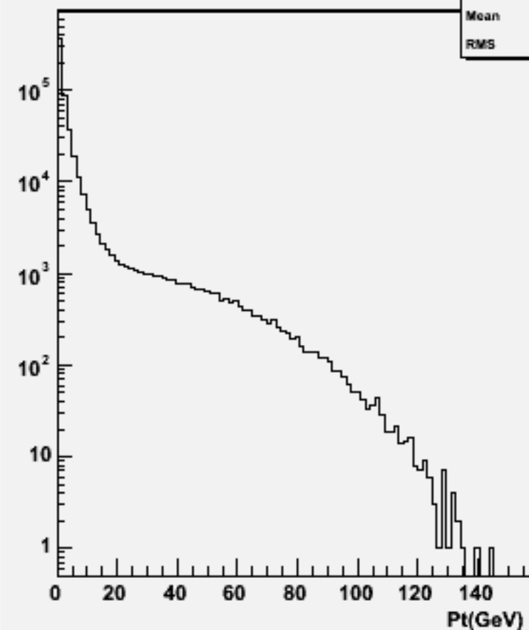
Particle Pt : w101198 bbn1e1e1n1_o
