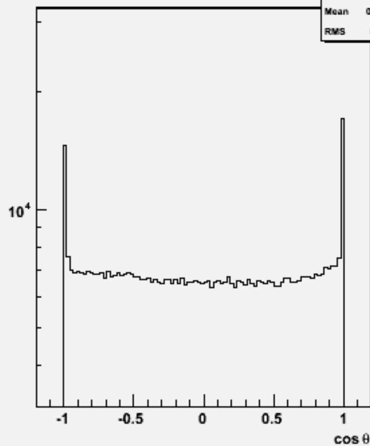
Particle cos \theta : w101196 bbn1e1e1n1_o
