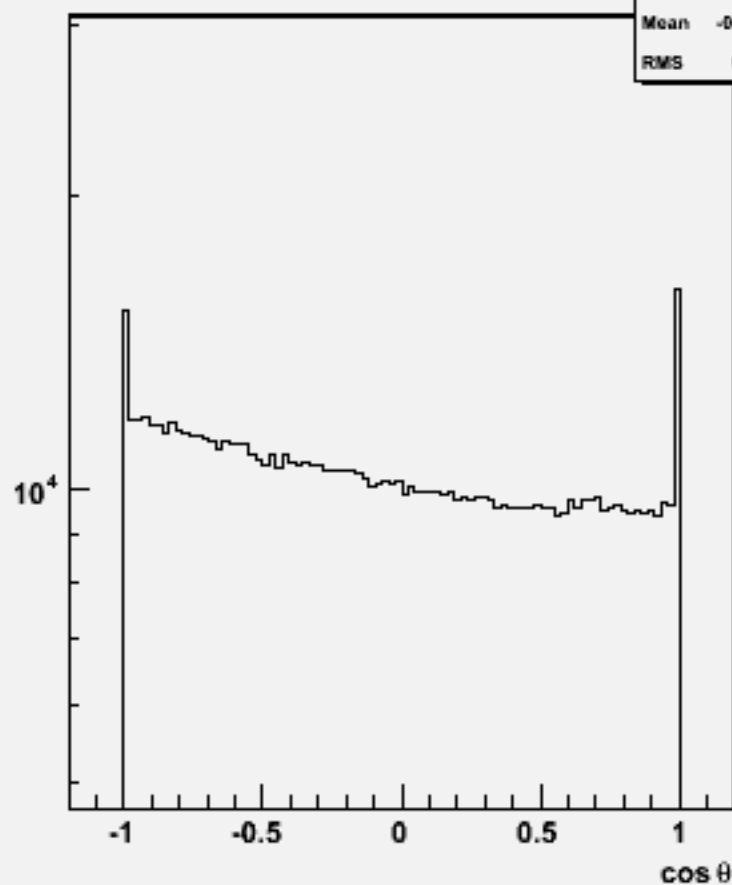
Particle \cos\theta : w101185 sscse3n3_o
