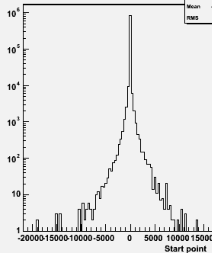
Start point Z : w101185 sscse3n3_o
