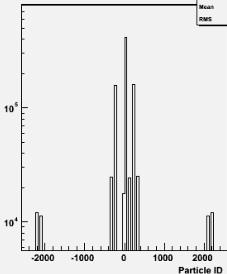
Particle ID : w101185 sscse3n3_o
