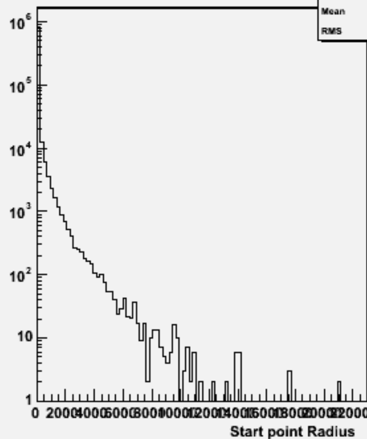
Start point R : w101185 sscse3n3_o
