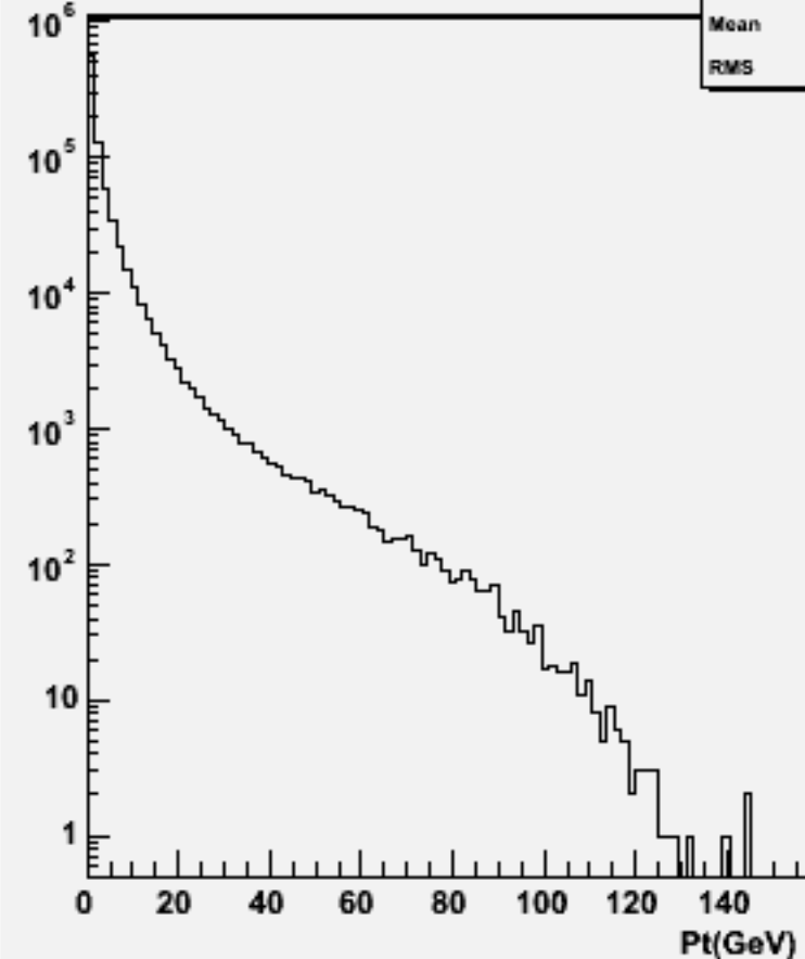
Particle Pt : w101185 sscse3n3_o
