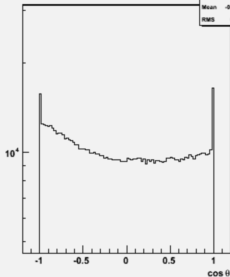
Particle cosθ : w101180 sscse2n2_o
