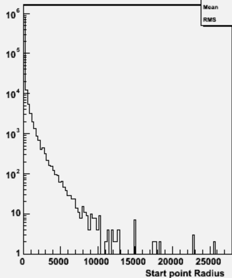
Start point R : w101180 sscse2n2_o
