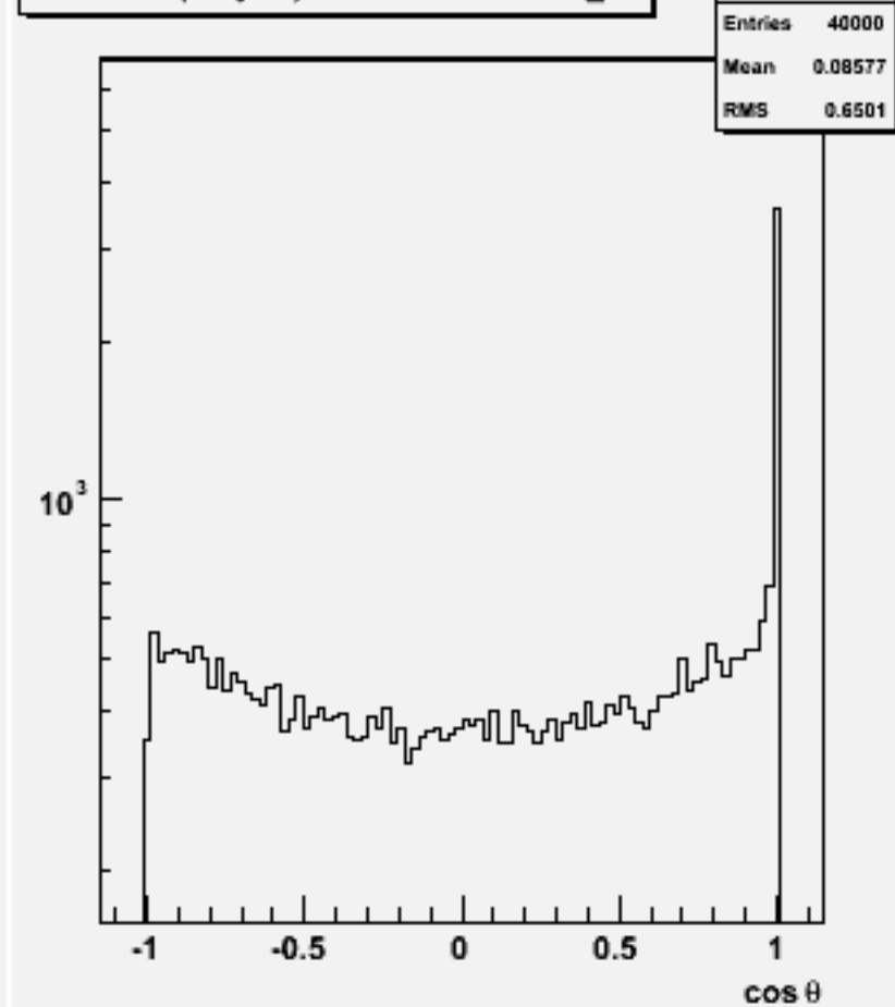
Jet cosθ (All jets)w101180 sscse2n2_o
