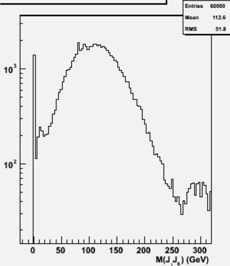
2jets mass(All comb)w101180 sscse2n2_o
