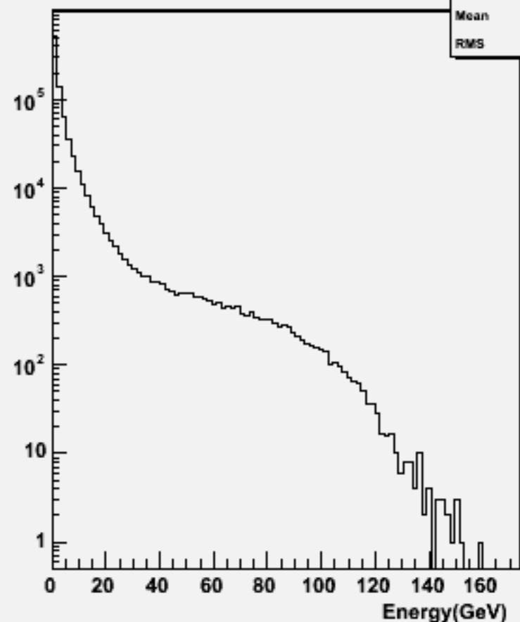
Particle Energy : w101180 sscse2n2_o
