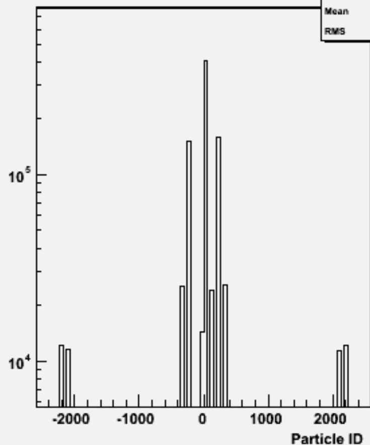
Particle ID : w101180 sscse2n2_o
