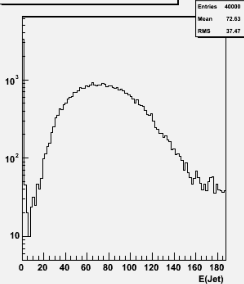
Jet energies(All jets)w101180 sscse2n2_o
