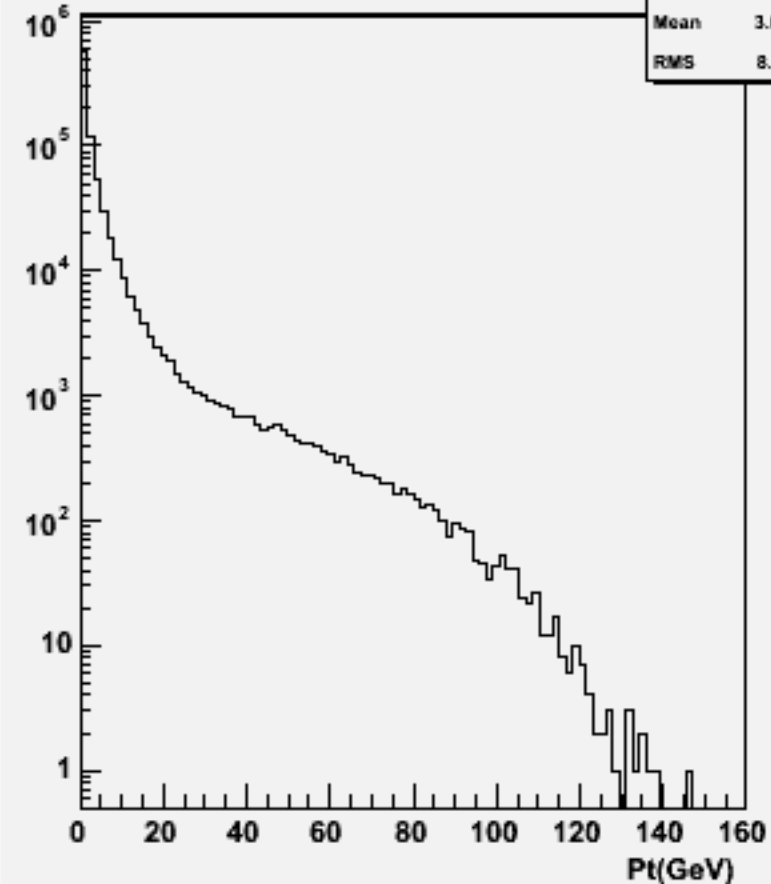
Particle Pt : w101180 sscse2n2_o
