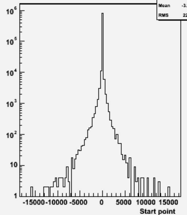
Start point Z : w101180 sscse2n2_o
