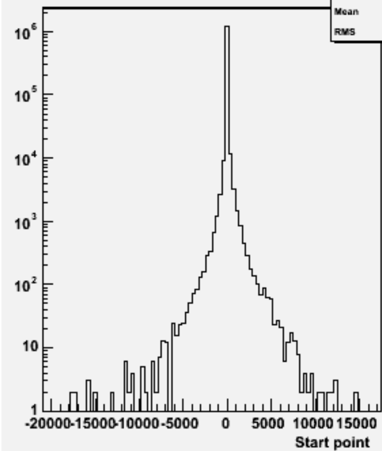
Start point Z : w101172 ssudsc_o
