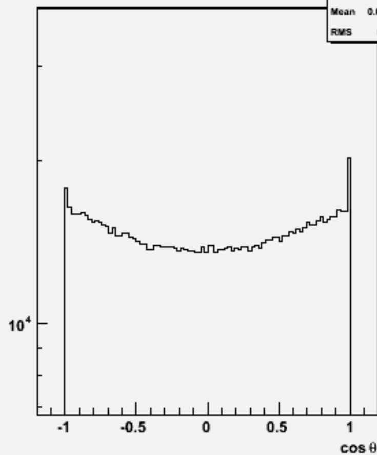
Particle cosθ : w101172 ssudsc_o
