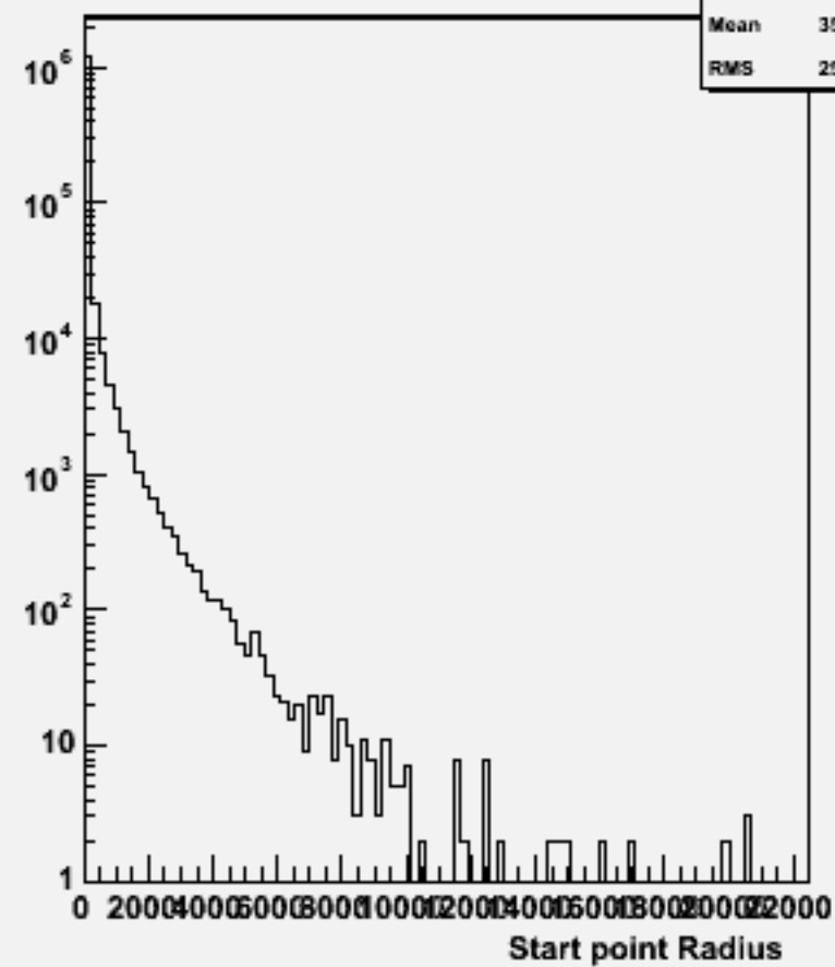
Start point R : w101172 ssudsc_o
