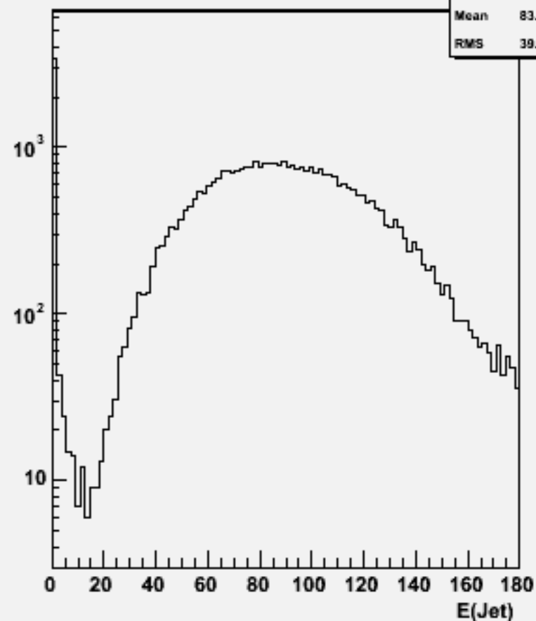
Jet energies(All jets)w101172 ssudsc_o
