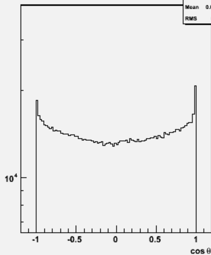
Particle cos \theta : w101169 ssuddu_o
