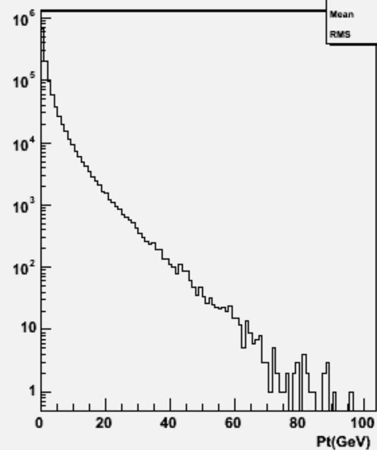
Particle Pt : w101169 ssuddu_o
