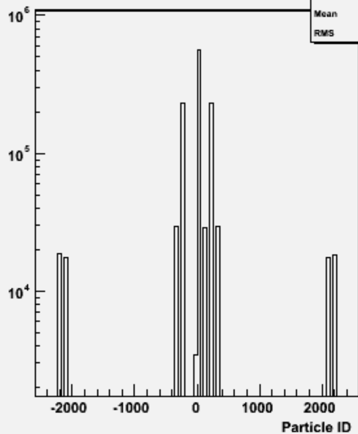
Particle ID : w101169 ssuddu_o
