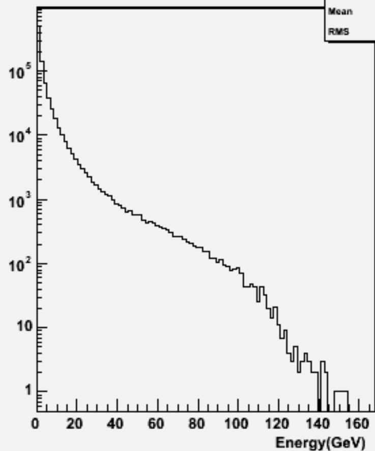
Particle Energy : w101165 ssude3n3_o
