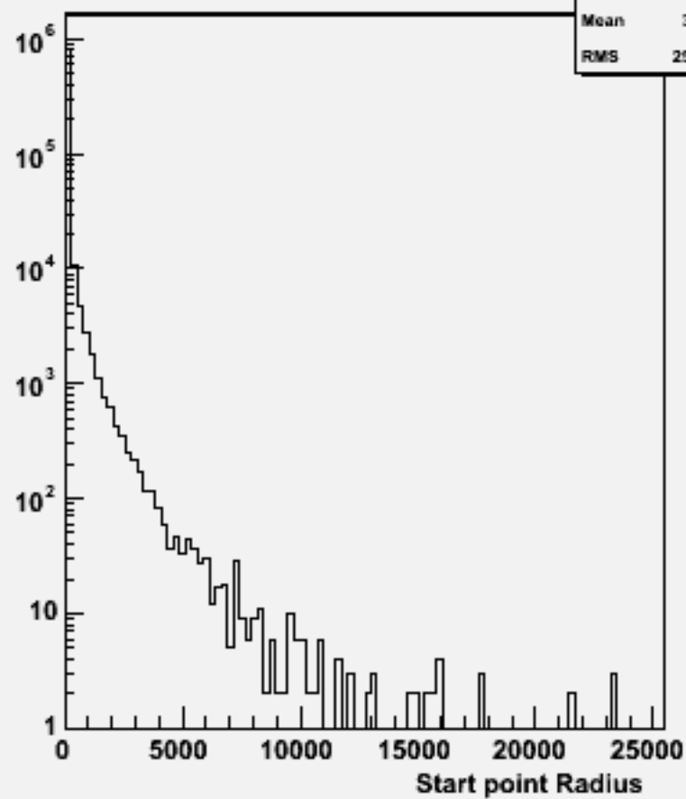
Start point R : w101165 ssude3n3_o
