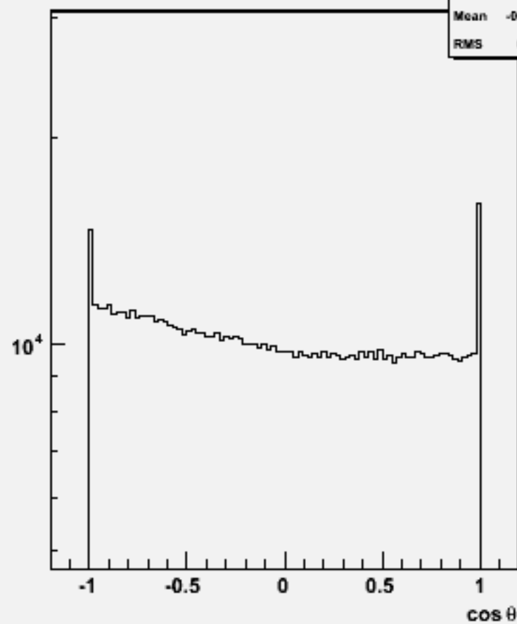
Particle cos \theta : w101165 ssude3n3_o
