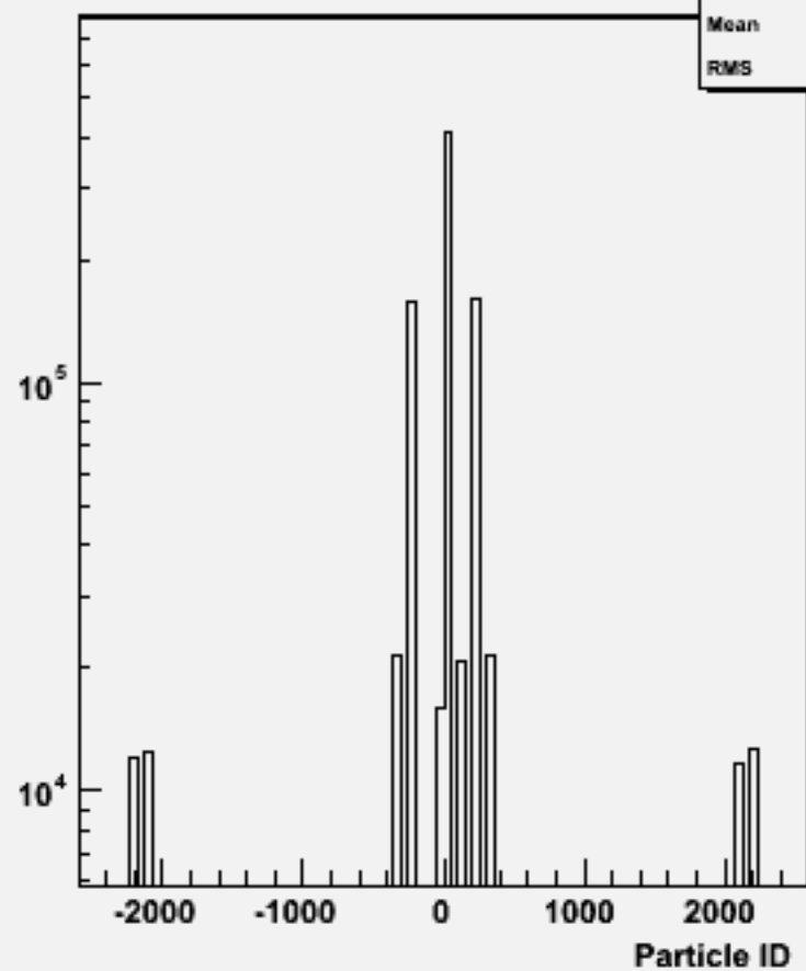
Particle ID : w101165 ssude3n3_o
