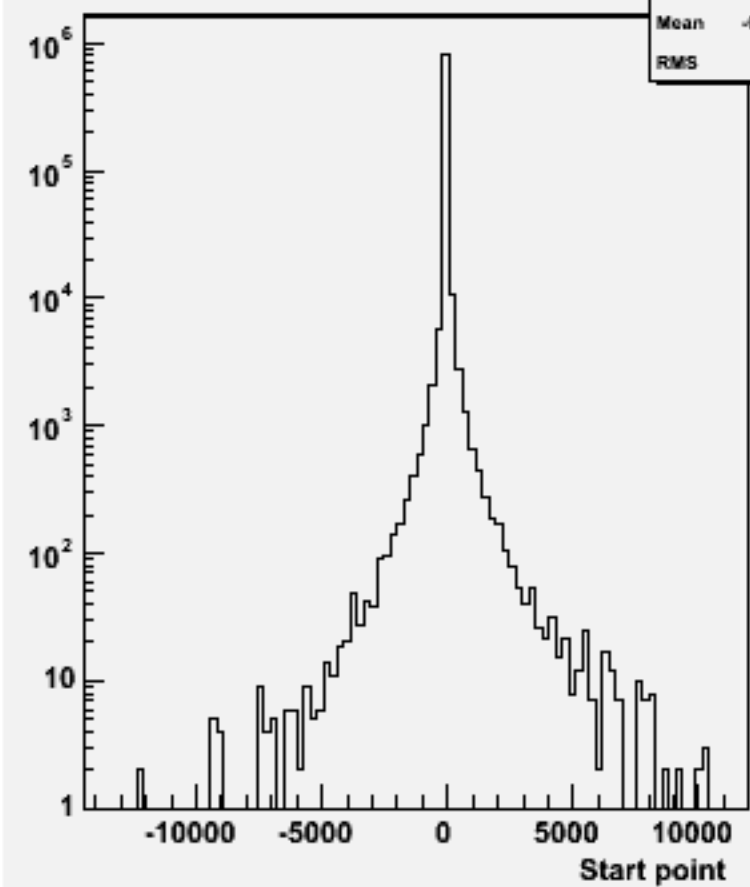
Start point Z : w101165 ssude3n3_o
