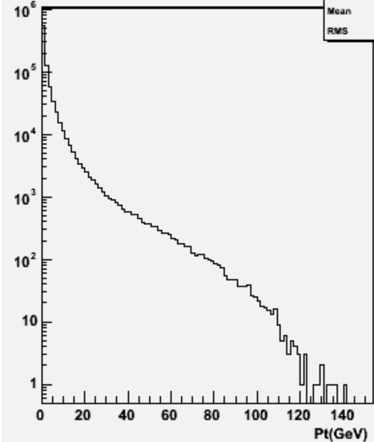
Particle Pt : w101165 ssude3n3_o
