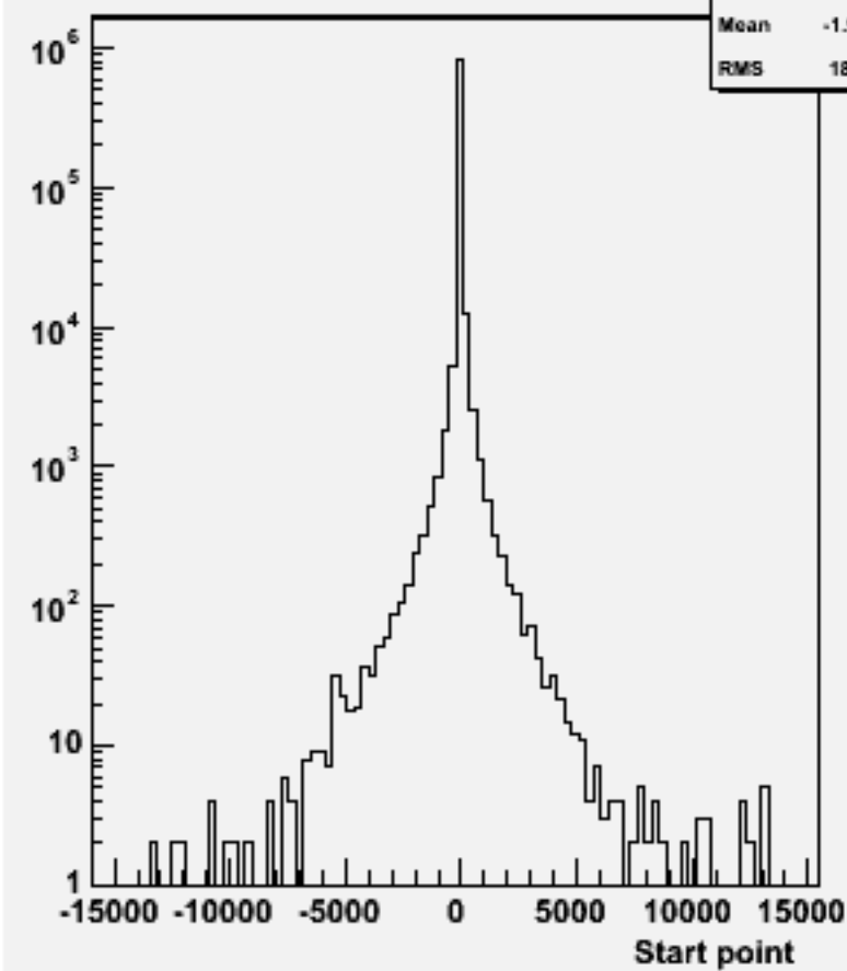
Start point Z : w101164 ssude3n3_o
