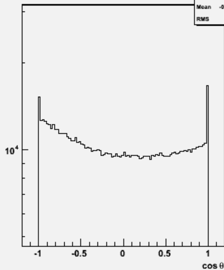
Particle cos \theta : w101164 ssude3n3_o
