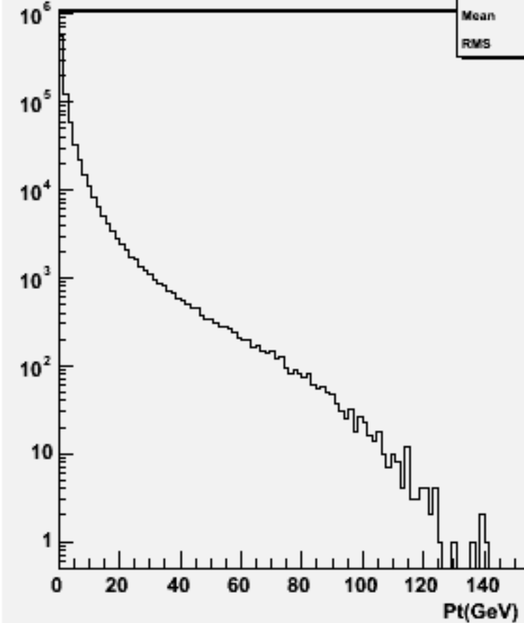
Particle Pt : w101164 ssude3n3_o
