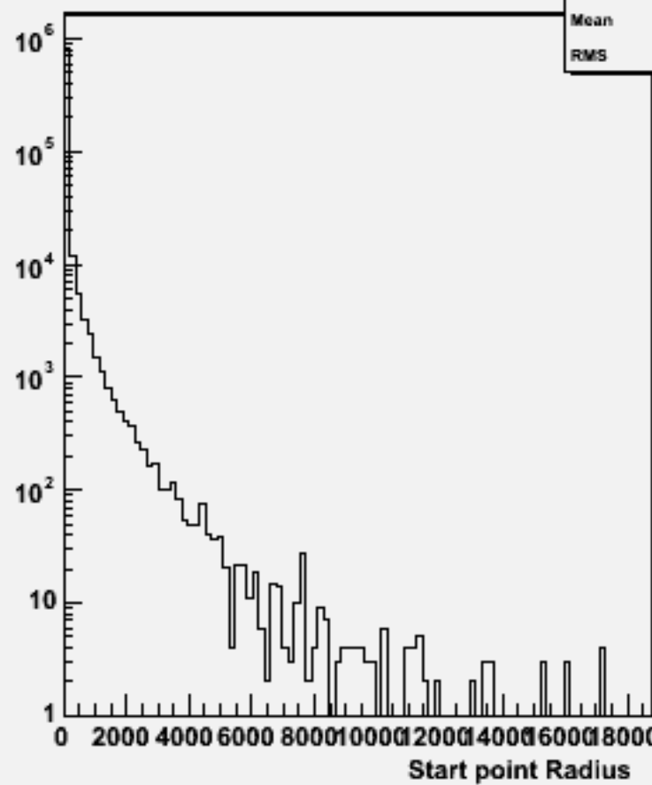
Start point R : w101164 ssude3n3_o
