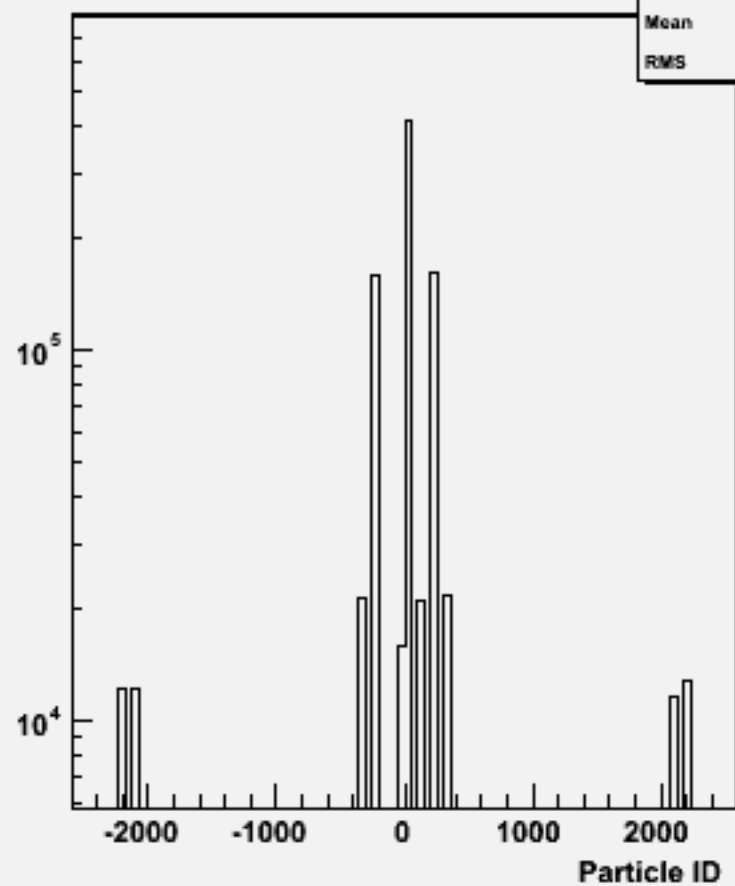
Particle ID : w101164 ssude3n3_o
