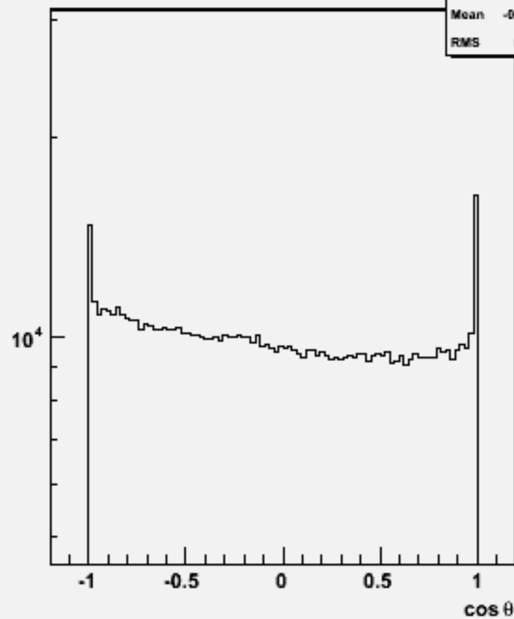
Particle cos \theta : w101161 ssude2n2_o
