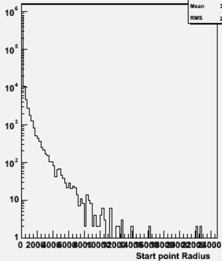
Start point R : w101161 ssude2n2_o
