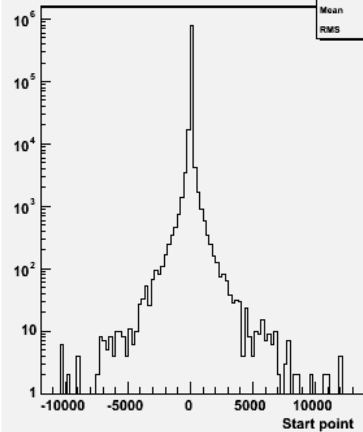
Start point Z : w101161 ssude2n2_o
