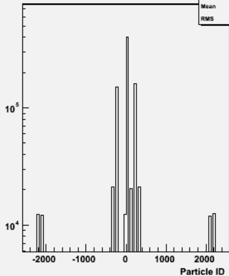
Particle ID : w101161 ssude2n2_o
